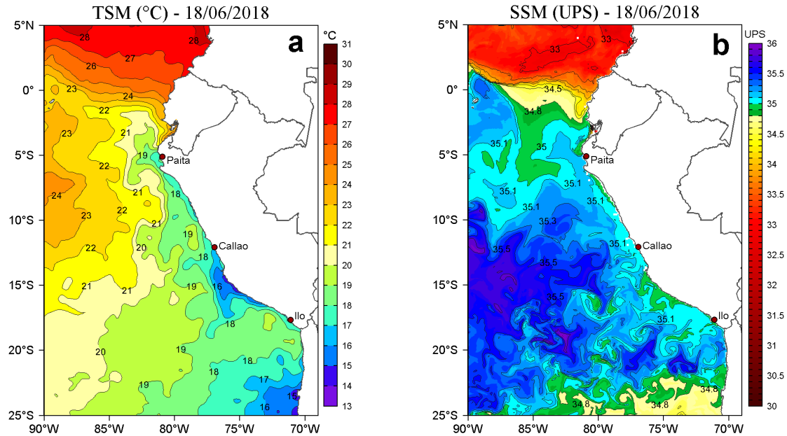
Figura 2. a) Temperatura Superficial del Mar ( ^{\circ}\text{C} ) y b) Salinidad Superficial del Mar (UPS) para el 18 de junio de 2018. Datos: OSTIA-UKMO-L4-GLOB-v2.0 (UK Met Office, 2012; Donlon et al, 2012) disponible en https://podaac.jpl.nasa.gov/dataset/OSTIA-UKMO-L4-GLOB-v2.0 para (a) y Hybrid Coordinate Ocean Model (HYCOM; Halliwell et al., 1998; 2000; Bleck, 2001) para (b). Procesamiento: LHF/AFIOF/DGIOCC/IMARPE.
