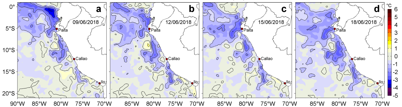
Figura 3. Anomalías de la Temperatura Superficial del Mar ( ^{\circ}\text{C} ) para los días: a) 09, b) 12, c) 15 y d) 18 de junio de 2018. Las anomalías se calcularon respecto de la climatología para el periodo 2007-2016. Datos: OSTIA-UKMO-L4-GLOB-v2.0 (UK Met Office, 2012; Donlon et al, 2012). Procesamiento: LHF/AFIOF/DGIOCC/IMARPE.
