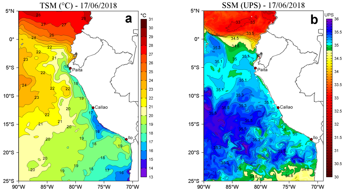
Figura 2. a) Temperatura Superficial del Mar ( ^{\circ}\text{C} ) y b) Salinidad Superficial del Mar (UPS) para el 17 de junio de 2018. Datos: OSTIA-UKMO-L4-GLOB-v2.0 (UK Met Office, 2012; Donlon et al, 2012) disponible en https://podaac.jpl.nasa.gov/dataset/OSTIA-UKMO-L4-GLOB-v2.0 para (a) y Hybrid Coordinate Ocean Model (HYCOM; Halliwell et al., 1998; 2000; Bleck, 2001) para (b). Procesamiento: LHFM/AFIOF/DGIOCC/IMARPE.
