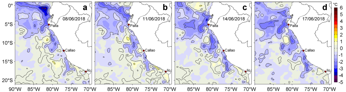
Figura 3. Anomalías de la Temperatura Superficial del Mar ( ^{\circ}\text{C} ) para los días: a) 08, b) 11, c) 14 y d) 17 de junio de 2018. Las anomalías se calcularon respecto de la climatología para el periodo 2007-2016. Datos: OSTIA-UKMO-L4-GLOB-v2.0 (UK Met Office, 2012; Donlon et al, 2012). Procesamiento: LHFM/AFIOF/DGIOCC/IMARPE.
