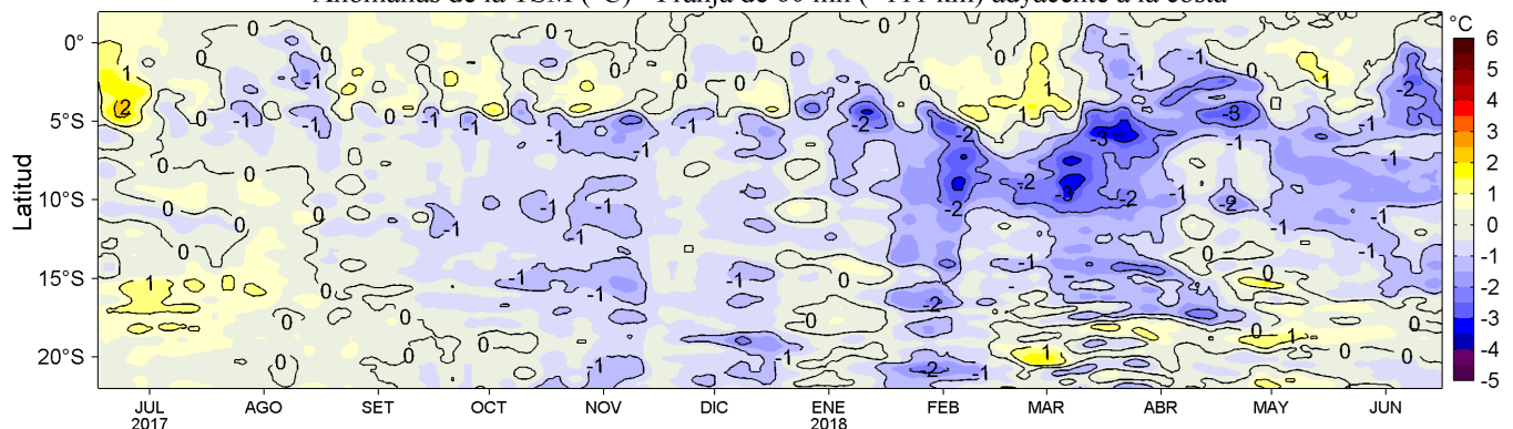
Figura 4. Variación promedio de las anomalías de la Temperatura Superficial del Mar (°C) para una franja de 60 mn (~111 km) adyacente al litoral peruano para los últimos doce meses al 16 de junio de 2018. Datos: OSTIA-UKMO-L4-GLOB-v2.0 (UK Met. Office, 2012; Donlon et al, 2012) disponible en https://podaac.jpl.nasa.gov/dataset/OSTIA-UKMO-L4-GLOB-v2.0 . Las anomalías se calcularon con respecto al periodo 2007-2016. Procesamiento: LHF/AFIOF/DGIOCC/IMARPE.
