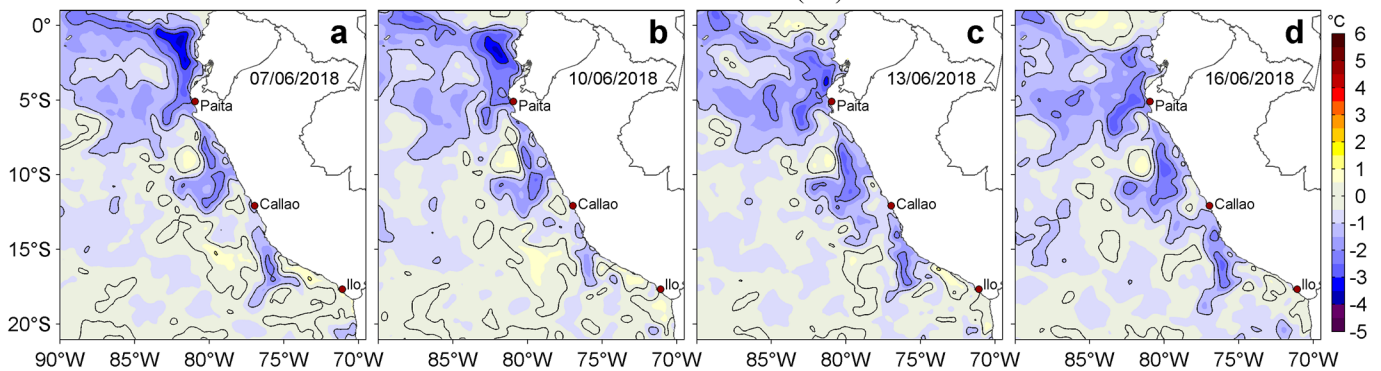
Figura 3. Anomalías de la Temperatura Superficial del Mar (°C) para los días: a) 07, b) 10, c) 13 y d) 16 de junio de 2018. Las anomalías se calcularon respecto de la climatología para el periodo 2007-2016. Datos: OSTIA-UKMO-L4-GLOB-v2.0 (UK Met Office, 2012; Donlon et al, 2012). Procesamiento: LHF/AFIOF/DGIOCC/IMARPE.
