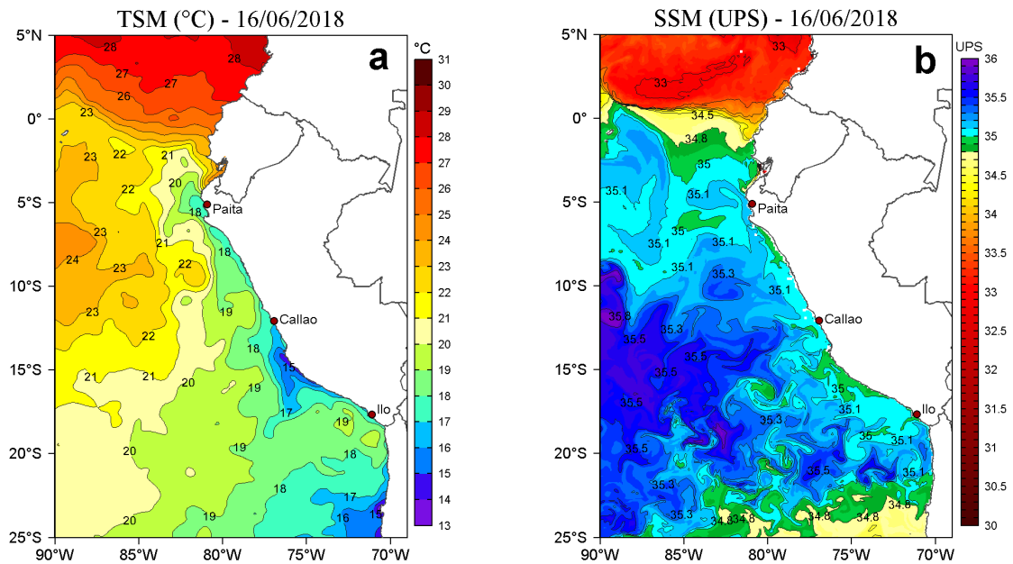
Figura 2. a) Temperatura Superficial del Mar (°C) y b) Salinidad Superficial del Mar (UPS) para el 16 de junio de 2018. Datos: OSTIA-UKMO-L4-GLOB-v2.0 (UK Met Office, 2012; Donlon et al, 2012) disponible en https://podaac.jpl.nasa.gov/dataset/OSTIA-UKMO-L4-GLOB-v2.0 para (a) y Hybrid Coordinate Ocean Model (HYCOM; Halliwell et al., 1998; 2000; Bleck, 2001) para (b). Procesamiento: LHF/AFIOF/DGIOCC/IMARPE.
