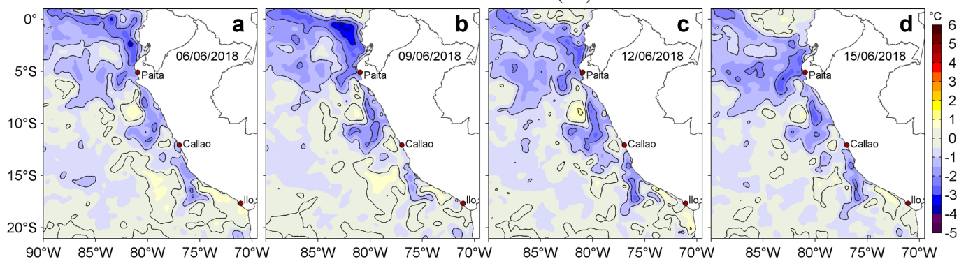
Figura 3. Anomalías de la Temperatura Superficial del Mar (°C) para los días: a) 06, b) 09, c) 12 y d) 15 de junio de 2018. Las anomalías se calcularon respecto de la climatología para el periodo 2007-2016. Datos: OSTIA-UKMO-L4-GLOB-v2.0 (UK Met Office, 2012; Donlon et al, 2012). Procesamiento: LHFM/AFIOF/DGIOCC/IMARPE.
