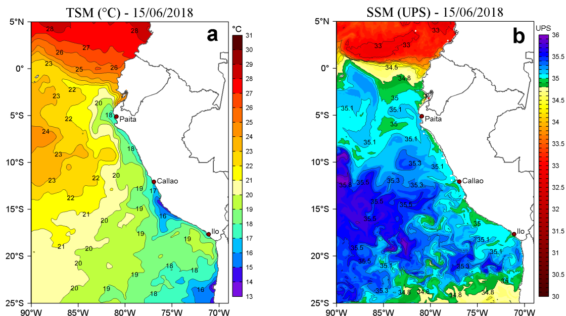
Figura 2. a) Temperatura Superficial del Mar (°C) y b) Salinidad Superficial del Mar (UPS) para el 15 de junio de 2018. Datos: OSTIA-UKMO-L4-GLOB-v2.0 (UK Met Office, 2012; Donlon et al, 2012) disponible en https://podaac.jpl.nasa.gov/dataset/OSTIA-UKMO-L4-GLOB-v2.0 para (a) y Hybrid Coordinate Ocean Model (HYCOM; Halliwell et al., 1998; 2000; Bleck, 2001) para (b). Procesamiento: LHFM/AFIOF/DGIOCC/IMARPE.
