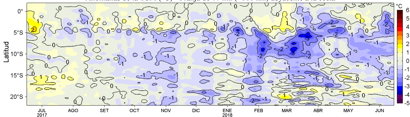
Figura 4. Variación promedio de las anomalías de la Temperatura Superficial del Mar (°C) para una franja de 60 mn (~111 km) adyacente al litoral peruano para los últimos doce meses al 15 de junio de 2018. Datos: OSTIA-UKMO-L4-GLOB-v2.0 (UK Met. Office, 2012; Donlon et al, 2012) disponible en https://podaac.jpl.nasa.gov/dataset/OSTIA-UKMO-L4-GLOB-v2.0 . Las anomalías se calcularon con respecto al periodo 2007-2016. Procesamiento: LHFM/AFIOF/DGIOCC/IMARPE.
