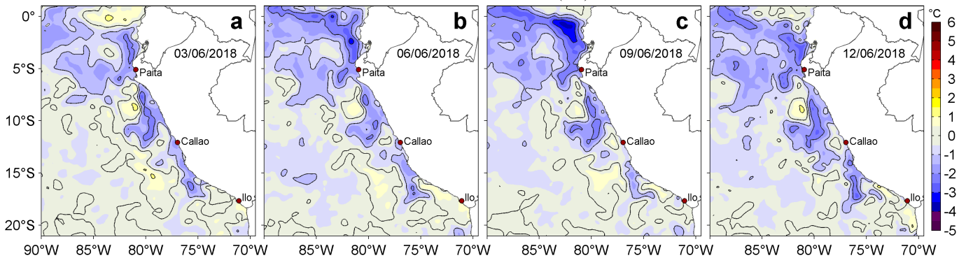
Figura 3. Anomalías de la Temperatura Superficial del Mar ( ^{\circ}\text{C} ) para los días: a) 03, b) 06, c) 09 y d) 12 de junio de 2018. Las anomalías se calcularon respecto de la climatología para el periodo 2007-2016. Datos: OSTIA-UKMO-L4-GLOB-v2.0 (UK Met Office, 2012; Donlon et al, 2012). Procesamiento: LHFM/AFIOF/DGIOCC/IMARPE.
