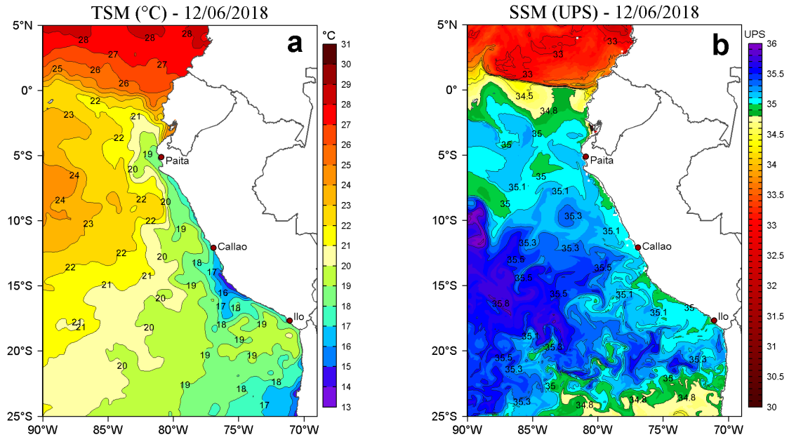
Figura 2. a) Temperatura Superficial del Mar ( ^{\circ}\text{C} ) y b) Salinidad Superficial del Mar (UPS) para el 12 de junio de 2018. Datos: OSTIA-UKMO-L4-GLOB-v2.0 (UK Met Office, 2012; Donlon et al, 2012) disponible en https://podaac.jpl.nasa.gov/dataset/OSTIA-UKMO-L4-GLOB-v2.0 para (a) y Hybrid Coordinate Ocean Model (HYCOM; Halliwell et al., 1998; 2000; Bleck, 2001) para (b). Procesamiento: LHFM/AFIOF/DGIOCC/IMARPE.
