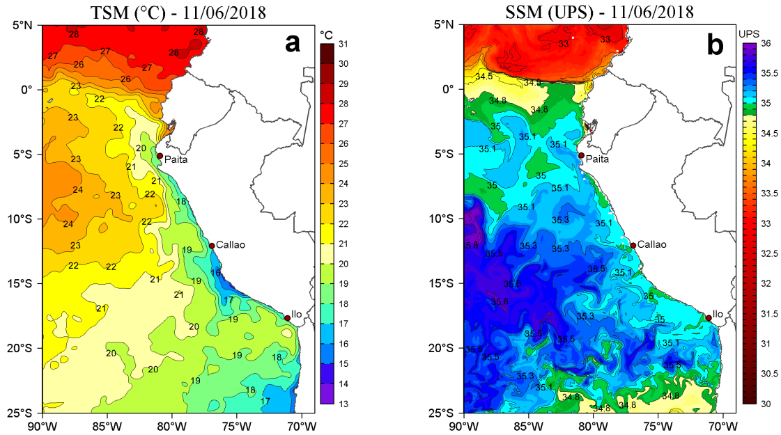
Figura 2. a) Temperatura Superficial del Mar ( ^{\circ}\text{C} ) y b) Salinidad Superficial del Mar (UPS) para el 11 de junio de 2018. Datos: OSTIA-UKMO-L4-GLOB-v2.0 (UK Met Office, 2012; Donlon et al, 2012) disponible en https://podaac.jpl.nasa.gov/dataset/OSTIA-UKMO-L4-GLOB-v2.0 para (a) y Hybrid Coordinate Ocean Model (HYCOM; Halliwell et al., 1998; 2000; Bleck, 2001) para (b). Procesamiento: LHF/AFIOF/DGIOCC/IMARPE.
