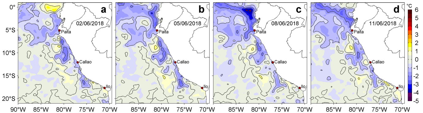
Figura 3. Anomalías de la Temperatura Superficial del Mar ( ^{\circ}\text{C} ) para los días: a) 02, b) 05, c) 08 y d) 11 de junio de 2018. Las anomalías se calcularon respecto de la climatología para el periodo 2007-2016. Datos: OSTIA-UKMO-L4-GLOB-v2.0 (UK Met Office, 2012; Donlon et al, 2012). Procesamiento: LHF/AFIOF/DGIOCC/IMARPE.
