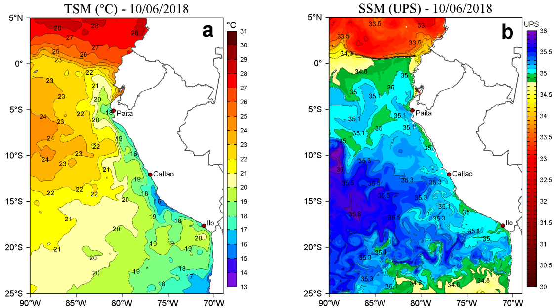
Figura 2. a) Temperatura Superficial del Mar ( ^{\circ}\text{C} ) y b) Salinidad Superficial del Mar (UPS) para el 10 de junio de 2018. Datos: OSTIA-UKMO-L4-GLOB-v2.0 (UK Met Office, 2012; Donlon et al, 2012) disponible en https://podaac.jpl.nasa.gov/dataset/OSTIA-UKMO-L4-GLOB-v2.0 para (a) y Hybrid Coordinate Ocean Model (HYCOM; Halliwell et al., 1998; 2000; Bleck, 2001) para (b). Procesamiento: LHF/AFIOF/DGIOCC/IMARPE.
