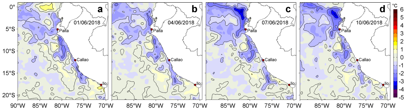
Figura 3. Anomalías de la Temperatura Superficial del Mar ( ^{\circ}\text{C} ) para los días: a) 01, b) 04, c) 07 y d) 10 de junio de 2018. Las anomalías se calcularon respecto de la climatología para el periodo 2007-2016. Datos: OSTIA-UKMO-L4-GLOB-v2.0 (UK Met Office, 2012; Donlon et al, 2012). Procesamiento: LHF/AFIOF/DGIOCC/IMARPE.
