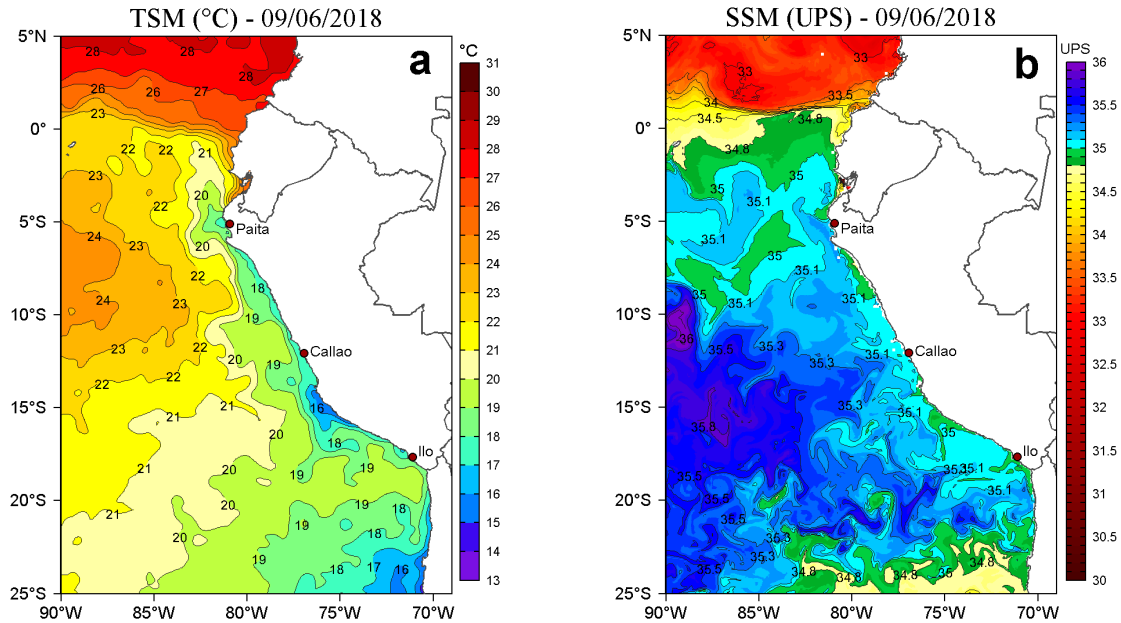
Figura 2. a) Temperatura Superficial del Mar ( ^{\circ}\text{C} ) y b) Salinidad Superficial del Mar (UPS) para el 09 de junio de 2018. Datos: OSTIA-UKMO-L4-GLOB-v2.0 (UK Met Office, 2012; Donlon et al, 2012) disponible en https://podaac.jpl.nasa.gov/dataset/OSTIA-UKMO-L4-GLOB-v2.0 para (a) y Hybrid Coordinate Ocean Model (HYCOM; Halliwell et al., 1998; 2000; Bleck, 2001) para (b). Procesamiento: LHF/AFIOF/DGIOCC/IMARPE.
