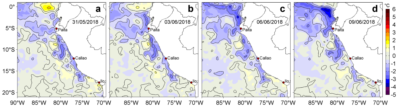
Figura 3. Anomalías de la Temperatura Superficial del Mar ( ^{\circ}\text{C} ) para los días: a) 31 de mayo, b) 03, c) 06 y d) 09 de junio de 2018. Las anomalías se calcularon respecto de la climatología para el periodo 2007-2016. Datos: OSTIA-UKMO-L4-GLOB-v2.0 (UK Met Office, 2012; Donlon et al, 2012). Procesamiento: LHF/AFIOF/DGIOCC/IMARPE.
