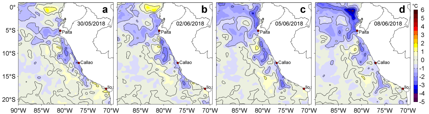
Figura 3. Anomalías de la Temperatura Superficial del Mar (°C) para los días: a) 30 de mayo, b) 02, c) 05 y d) 08 de junio de 2018. Las anomalías se calcularon respecto de la climatología para el periodo 2007-2016. Datos: OSTIA-UKMO-L4-GLOB-v2.0 (UK Met Office, 2012; Donlon et al, 2012). Procesamiento: LHF/AFIOF/DGIOCC/IMARPE.
