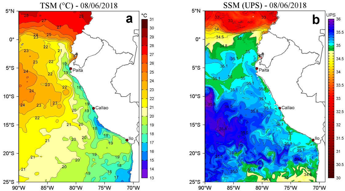
Figura 2. a) Temperatura Superficial del Mar (°C) y b) Salinidad Superficial del Mar (UPS) para el 08 de junio de 2018. Datos: OSTIA-UKMO-L4-GLOB-v2.0 (UK Met Office, 2012; Donlon et al, 2012) disponible en https://podaac.jpl.nasa.gov/dataset/OSTIA-UKMO-L4-GLOB-v2.0 para (a) y Hybrid Coordinate Ocean Model (HYCOM; Halliwell et al., 1998; 2000; Bleck, 2001) para (b). Procesamiento: LHF/AFIOF/DGIOCC/IMARPE.
