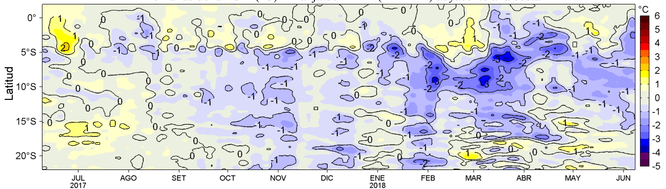
Figura 4. Variación promedio de las anomalías de la Temperatura Superficial del Mar (°C) para una franja de 60 mn (~111 km) adyacente al litoral peruano para los últimos doce meses al 08 de junio de 2018. Datos: OSTIA-UKMO-L4-GLOB-v2.0 (UK Met. Office, 2012; Donlon et al, 2012) disponible en https://podaac.jpl.nasa.gov/dataset/OSTIA-UKMO-L4-GLOB-v2.0 . Las anomalías se calcularon con respecto al periodo 2007-2016. Procesamiento: LHF/AFIOF/DGIOCC/IMARPE.
