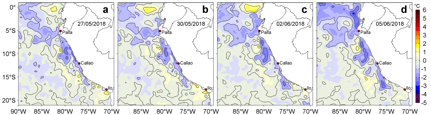
Figura 3. Anomalías de la Temperatura Superficial del Mar ( ^{\circ}\text{C} ) para los días: a) 27 y b) 30 de mayo, c) 02 y d) 05 de junio de 2018. Las anomalías se calcularon respecto de la climatología para el periodo 2007-2016. Datos: OSTIA-UKMO-L4-GLOB-v2.0 (UK Met Office, 2012; Donlon et al, 2012). Procesamiento: LHF/AFIOF/DGIOCC/IMARPE.
