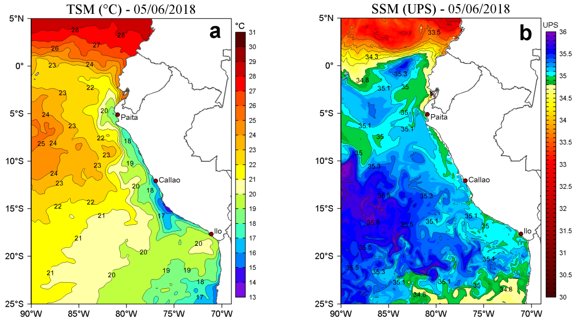
Figura 2. a) Temperatura Superficial del Mar ( ^{\circ}\text{C} ) y b) Salinidad Superficial del Mar (UPS) para el 05 de junio de 2018. Datos: OSTIA-UKMO-L4-GLOB-v2.0 (UK Met Office, 2012; Donlon et al, 2012) disponible en https://podaac.jpl.nasa.gov/dataset/OSTIA-UKMO-L4-GLOB-v2.0 para (a) y Hybrid Coordinate Ocean Model (HYCOM; Halliwell et al., 1998; 2000; Bleck, 2001) para (b). Procesamiento: LHF/AFIOF/DGIOCC/IMARPE.
