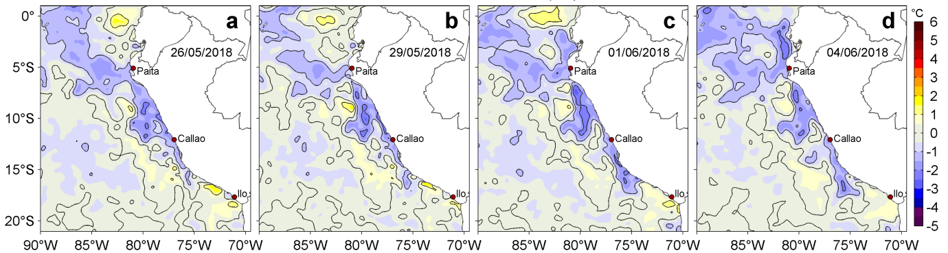
Figura 3. Anomalías de la Temperatura Superficial del Mar ( ^{\circ}\text{C} ) para los días: a) 26 y b) 29 de mayo, c) 01 y d) 04 de junio de 2018. Las anomalías se calcularon respecto de la climatología para el periodo 2007-2016. Datos: OSTIA-UKMO-L4-GLOB-v2.0 (UK Met Office, 2012; Donlon et al, 2012). Procesamiento: LHF/AFIOF/DGIOCC/IMARPE.
