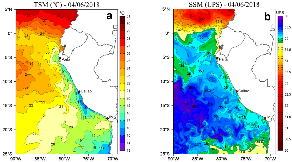
Figura 2. a) Temperatura Superficial del Mar ( ^{\circ}\text{C} ) y b) Salinidad Superficial del Mar (UPS) para el 04 de junio de 2018. Datos: OSTIA-UKMO-L4-GLOB-v2.0 (UK Met Office, 2012; Donlon et al, 2012) disponible en https://podaac.jpl.nasa.gov/dataset/OSTIA-UKMO-L4-GLOB-v2.0 para (a) y Hybrid Coordinate Ocean Model (HYCOM; Halliwell et al., 1998; 2000; Bleck, 2001) para (b). Procesamiento: LHF/AFIOF/DGIOCC/IMARPE.
