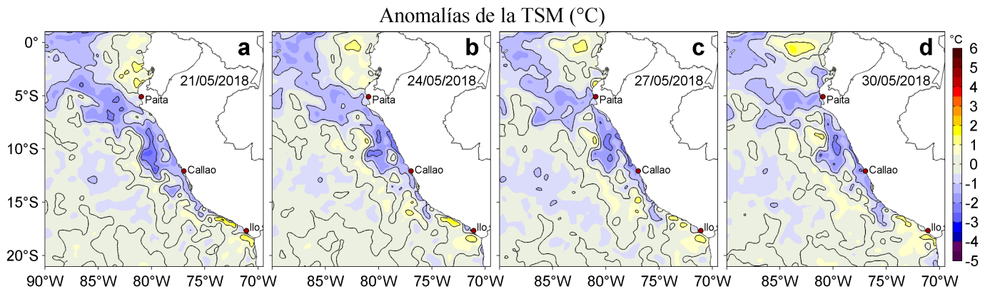
Figura 3. Anomalías de la Temperatura Superficial del Mar ( ^{\circ}\text{C} ) para los días: a) 21, b) 24, c) 27 y d) 30 de mayo de 2018. Las anomalías se calcularon respecto de la climatología para el periodo 2007-2016. Datos: OSTIA-UKMO-L4-GLOB-v2.0 (UK Met Office, 2012; Donlon et al, 2012). Procesamiento: LHF/AFIOF/DGIOCC/IMARPE.
