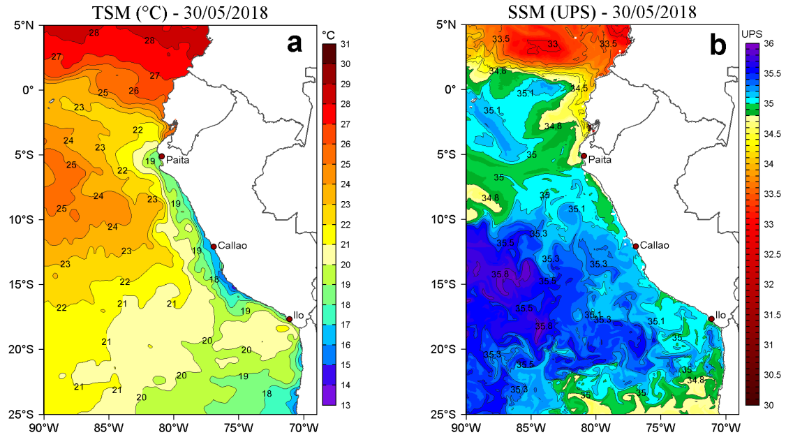
Figura 2. a) Temperatura Superficial del Mar ( ^{\circ}\text{C} ) y b) Salinidad Superficial del Mar (UPS) para el 30 de mayo de 2018. Datos: OSTIA-UKMO-L4-GLOB-v2.0 (UK Met Office, 2012; Donlon et al, 2012) disponible en https://podaac.jpl.nasa.gov/dataset/OSTIA-UKMO-L4-GLOB-v2.0 para (a) y Hybrid Coordinate Ocean Model (HYCOM; Halliwell et al., 1998; 2000; Bleck, 2001) para (b). Procesamiento: LHF/AFIOF/DGIOCC/IMARPE.
