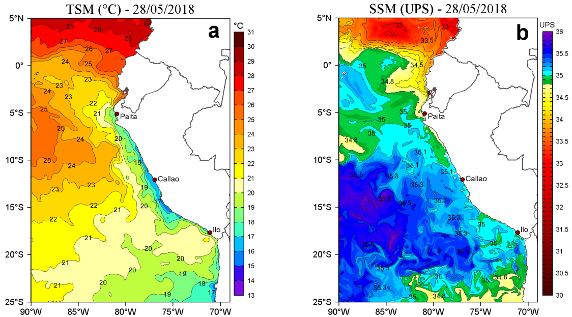
Figura 2. a) Temperatura Superficial del Mar ( ^{\circ}\text{C} ) y b) Salinidad Superficial del Mar (UPS) para el 28 de mayo de 2018. Datos: OSTIA-UKMO-L4-GLOB-v2.0 (UK Met Office, 2012; Donlon et al, 2012) disponible en https://podaac.jpl.nasa.gov/dataset/OSTIA-UKMO-L4-GLOB-v2.0 para (a) y Hybrid Coordinate Ocean Model (HYCOM; Halliwell et al., 1998; 2000; Bleck, 2001) para (b). Procesamiento: LHF/AFIOF/DGIOCC/IMARPE.
