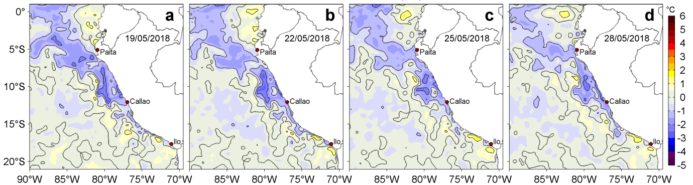
Figura 3. Anomalías de la Temperatura Superficial del Mar ( ^{\circ}\text{C} ) para los días: a) 19, b) 22, c) 25 y d) 28 de mayo de 2018. Las anomalías se calcularon respecto de la climatología para el periodo 2007-2016. Datos: OSTIA-UKMO-L4-GLOB-v2.0 (UK Met Office, 2012; Donlon et al, 2012). Procesamiento: LHF/AFIOF/DGIOCC/IMARPE.
