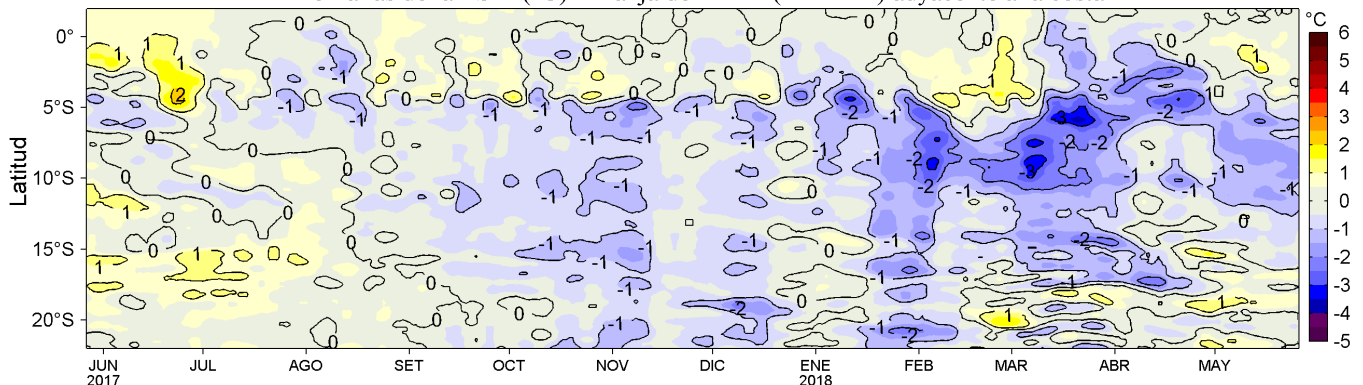
Figura 4. Variación promedio de las anomalías de la Temperatura Superficial del Mar (°C) para una franja de 60 mn (~111 km) adyacente al litoral peruano para los últimos doce meses al 26 de mayo de 2018. Datos: OSTIA-UKMO-L4-GLOB-v2.0 (UK Met. Office, 2012; Donlon et al, 2012) disponible en https://podaac.jpl.nasa.gov/dataset/OSTIA-UKMO-L4-GLOB-v2.0 . Las anomalías se calcularon con respecto al periodo 2007-2016. Procesamiento: LHF/AFIOF/DGIOCC/IMARPE.
