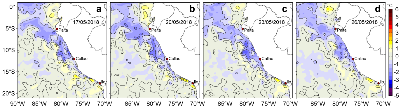
Figura 3. Anomalías de la Temperatura Superficial del Mar (°C) para los días: a) 17, b) 20, c) 23 y d) 26 de mayo de 2018. Las anomalías se calcularon respecto de la climatología para el periodo 2007-2016. Datos: OSTIA-UKMO-L4-GLOB-v2.0 (UK Met Office, 2012; Donlon et al, 2012). Procesamiento: LHF/AFIOF/DGIOCC/IMARPE.
