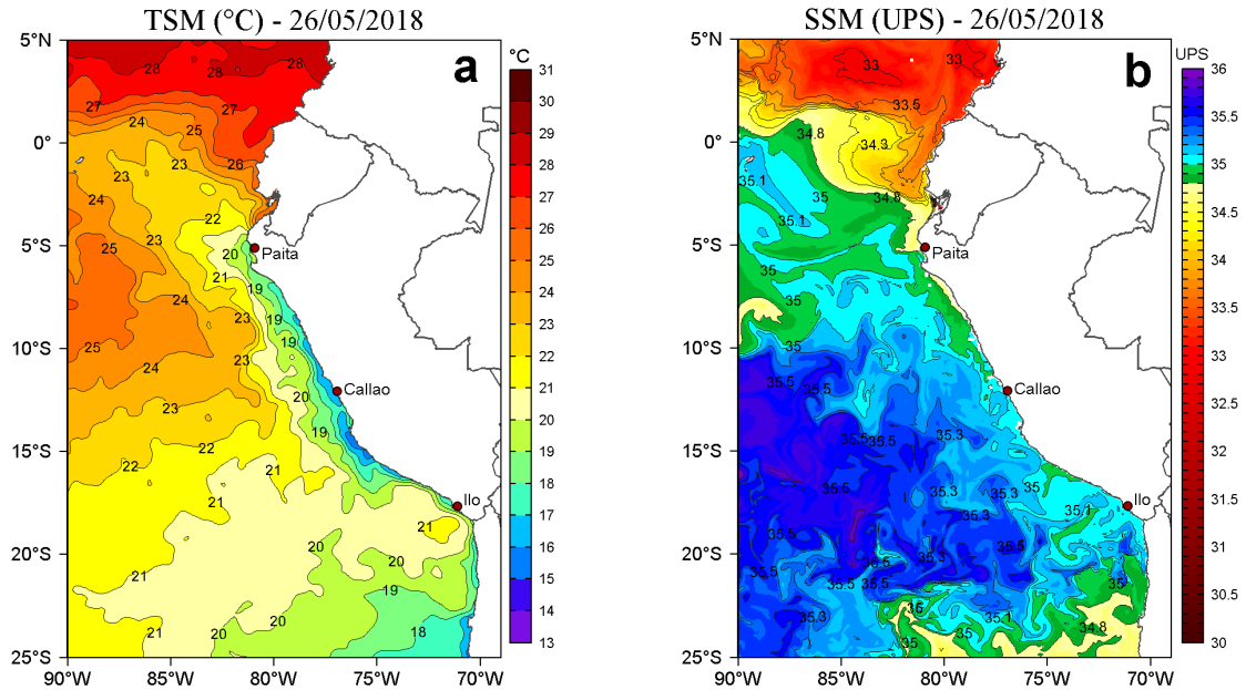
Figura 2. a) Temperatura Superficial del Mar (°C) y b) Salinidad Superficial del Mar (UPS) para el 26 de mayo de 2018. Datos: OSTIA-UKMO-L4-GLOB-v2.0 (UK Met Office, 2012; Donlon et al, 2012) disponible en https://podaac.jpl.nasa.gov/dataset/OSTIA-UKMO-L4-GLOB-v2.0 para (a) y Hybrid Coordinate Ocean Model (HYCOM; Halliwell et al., 1998; 2000; Bleck, 2001) para (b). Procesamiento: LHF/AFIOF/DGIOCC/IMARPE.
