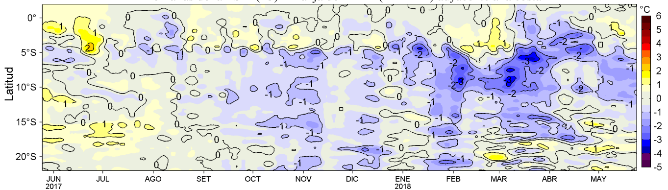
Figura 4. Variación promedio de las anomalías de la Temperatura Superficial del Mar (°C) para una franja de 60 mn (~111 km) adyacente al litoral peruano para los últimos doce meses al 24 de mayo de 2018. Datos: OSTIA-UKMO-L4-GLOB-v2.0 (UK Met. Office, 2012; Donlon et al, 2012) disponible en https://podaac.jpl.nasa.gov/dataset/OSTIA-UKMO-L4-GLOB-v2.0 . Las anomalías se calcularon con respecto al periodo 2007-2016. Procesamiento: LHF/AFIOF/DGIOCC/IMARPE.
