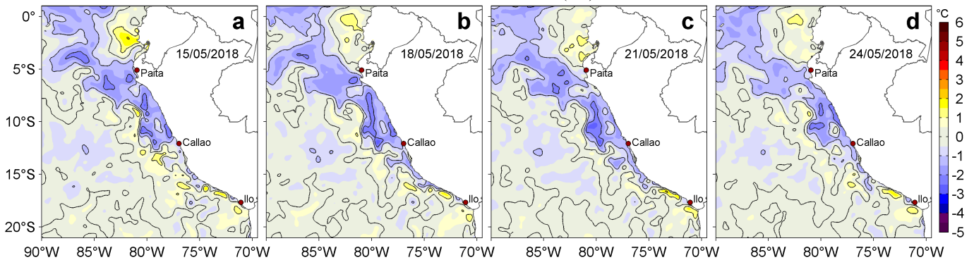
Figura 3. Anomalías de la Temperatura Superficial del Mar (°C) para los días: a) 15, b) 18, c) 21 y d) 24 de mayo de 2018. Las anomalías se calcularon respecto de la climatología para el periodo 2007-2016. Datos: OSTIA-UKMO-L4-GLOB-v2.0 (UK Met Office, 2012; Donlon et al, 2012). Procesamiento: LHF/AFIOF/DGIOCC/IMARPE.
