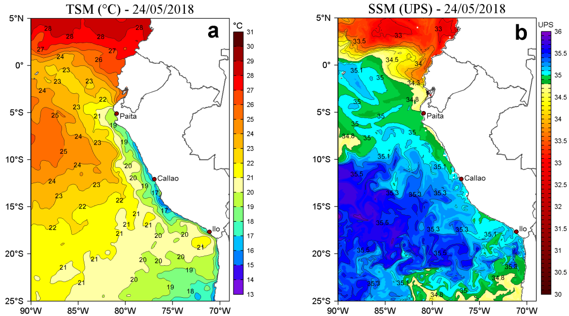
Figura 2. a) Temperatura Superficial del Mar (°C) y b) Salinidad Superficial del Mar (UPS) para el 24 de mayo de 2018. Datos: OSTIA-UKMO-L4-GLOB-v2.0 (UK Met Office, 2012; Donlon et al, 2012) disponible en https://podaac.jpl.nasa.gov/dataset/OSTIA-UKMO-L4-GLOB-v2.0 para (a) y Hybrid Coordinate Ocean Model (HYCOM; Halliwell et al., 1998; 2000; Bleck, 2001) para (b). Procesamiento: LHF/AFIOF/DGIOCC/IMARPE.
