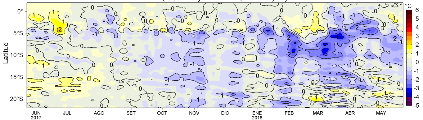
Figura 4. Variación promedio de las anomalías de la Temperatura Superficial del Mar (°C) para una franja de 60 mn (~111 km) adyacente al litoral peruano para los últimos doce meses al 22 de mayo de 2018. Datos: OSTIA-UKMO-L4-GLOB-v2.0 (UK Met. Office, 2012; Donlon et al, 2012) disponible en https://podaac.jpl.nasa.gov/dataset/OSTIA-UKMO-L4-GLOB-v2.0 . Las anomalías se calcularon con respecto al periodo 2007-2016. Procesamiento: LHF/AFIOF/DGIOCC/IMARPE.
