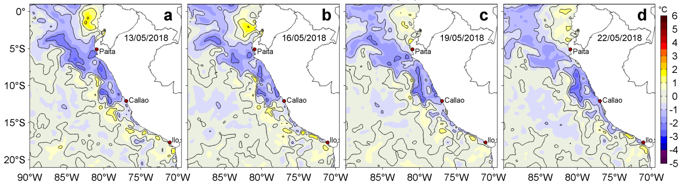
Figura 3. Anomalías de la Temperatura Superficial del Mar (°C) para los días: a) 13, b) 16, c) 19 y d) 22 de mayo de 2018. Las anomalías se calcularon respecto de la climatología para el periodo 2007-2016. Datos: OSTIA-UKMO-L4-GLOB-v2.0 (UK Met Office, 2012; Donlon et al, 2012). Procesamiento: LHF/AFIOF/DGIOCC/IMARPE.
