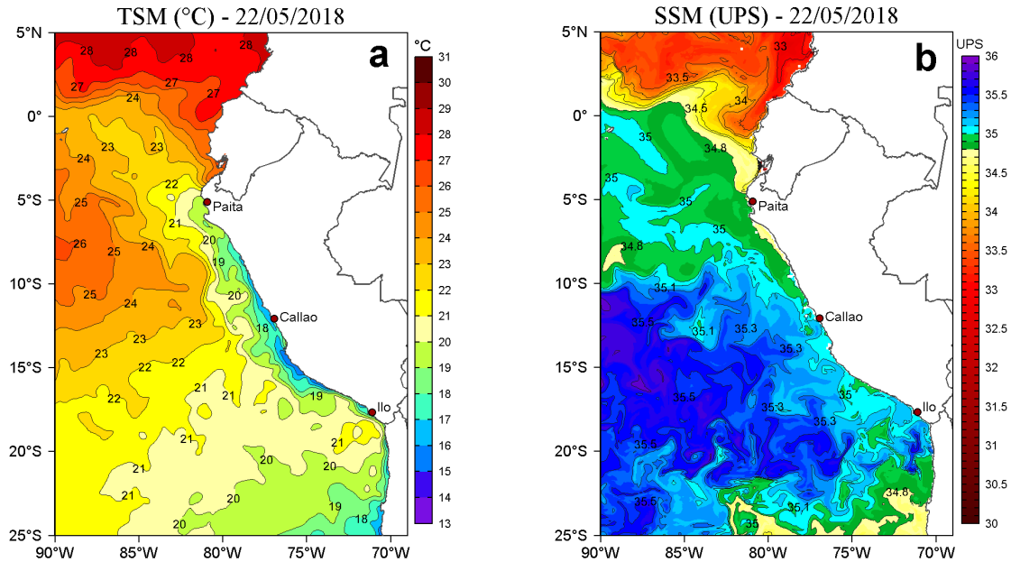
Figura 2. a) Temperatura Superficial del Mar (°C) y b) Salinidad Superficial del Mar (UPS) para el 22 de mayo de 2018. Datos: OSTIA-UKMO-L4-GLOB-v2.0 (UK Met Office, 2012; Donlon et al, 2012) disponible en https://podaac.jpl.nasa.gov/dataset/OSTIA-UKMO-L4-GLOB-v2.0 para (a) y Hybrid Coordinate Ocean Model (HYCOM; Halliwell et al., 1998; 2000; Bleck, 2001) para (b). Procesamiento: LHF/AFIOF/DGIOCC/IMARPE.
