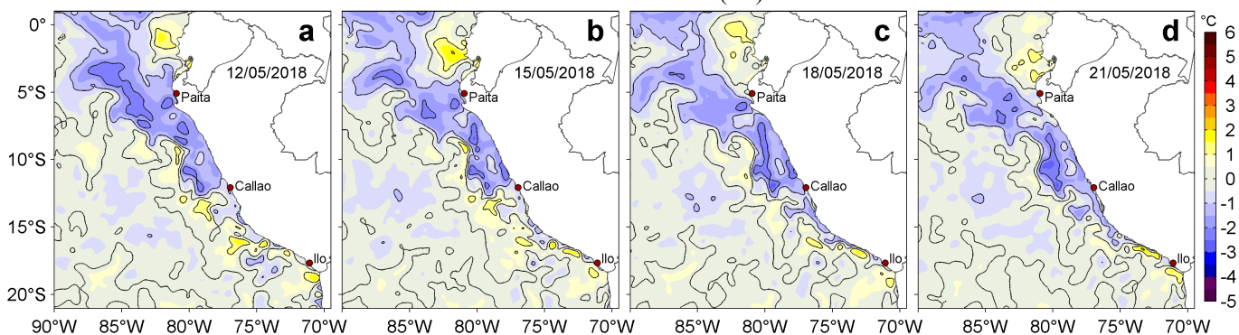
Figura 3. Anomalías de la Temperatura Superficial del Mar ( ^{\circ}\text{C} ) para los días: a) 12, b) 15, c) 18 y d) 21 de mayo de 2018. Las anomalías se calcularon respecto de la climatología para el periodo 2007-2016. Datos: OSTIA-UKMO-L4-GLOB-v2.0 (UK Met Office, 2012; Donlon et al, 2012). Procesamiento: LHF/AFIOF/DGIOCC/IMARPE.
