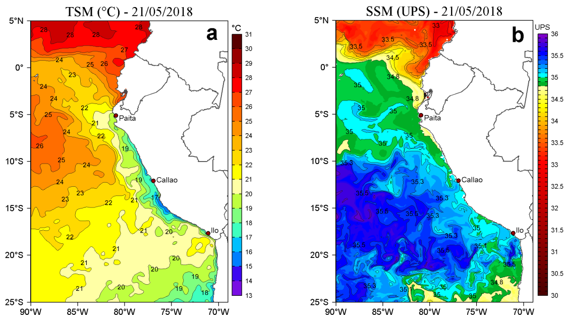
Figura 2. a) Temperatura Superficial del Mar ( ^{\circ}\text{C} ) y b) Salinidad Superficial del Mar (UPS) para el 21 de mayo de 2018. Datos: OSTIA-UKMO-L4-GLOB-v2.0 (UK Met Office, 2012; Donlon et al, 2012) disponible en https://podaac.jpl.nasa.gov/dataset/OSTIA-UKMO-L4-GLOB-v2.0 para (a) y Hybrid Coordinate Ocean Model (HYCOM; Halliwell et al., 1998; 2000; Bleck, 2001) para (b). Procesamiento: LHF/AFIOF/DGIOCC/IMARPE.
