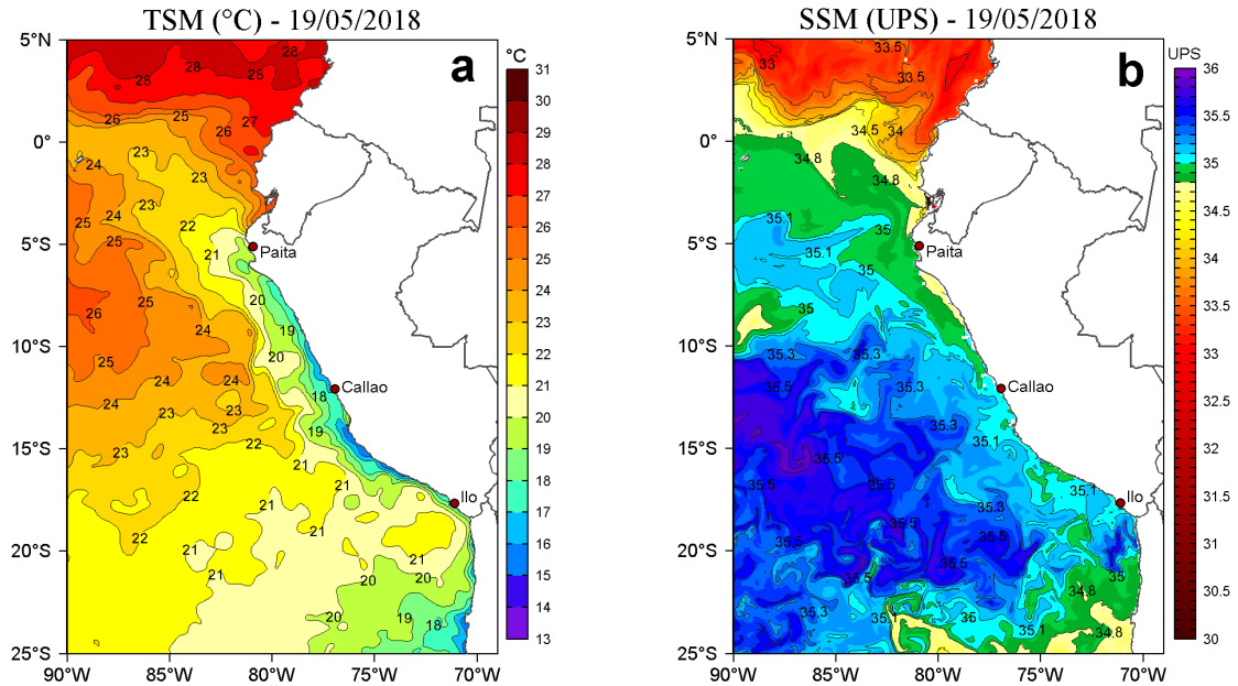
Figura 2. a) Temperatura Superficial del Mar (°C) y b) Salinidad Superficial del Mar (UPS) para el 19 de mayo de 2018. Datos: OSTIA-UKMO-L4-GLOB-v2.0 (UK Met Office, 2012; Donlon et al, 2012) disponible en https://podaac.jpl.nasa.gov/dataset/OSTIA-UKMO-L4-GLOB-v2.0 para (a) y Hybrid Coordinate Ocean Model (HYCOM; Halliwell et al., 1998; 2000; Bleck, 2001) para (b). Procesamiento: LHF/AFIOF/DGIOCC/IMARPE.
