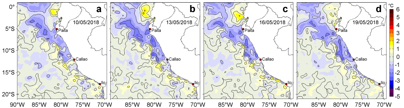
Figura 3. Anomalías de la Temperatura Superficial del Mar (°C) para los días: a) 10, b) 13, c) 16 y d) 19 de mayo de 2018. Las anomalías se calcularon respecto de la climatología para el periodo 2007-2016. Datos: OSTIA-UKMO-L4-GLOB-v2.0 (UK Met Office, 2012; Donlon et al, 2012). Procesamiento: LHF/AFIOF/DGIOCC/IMARPE.
