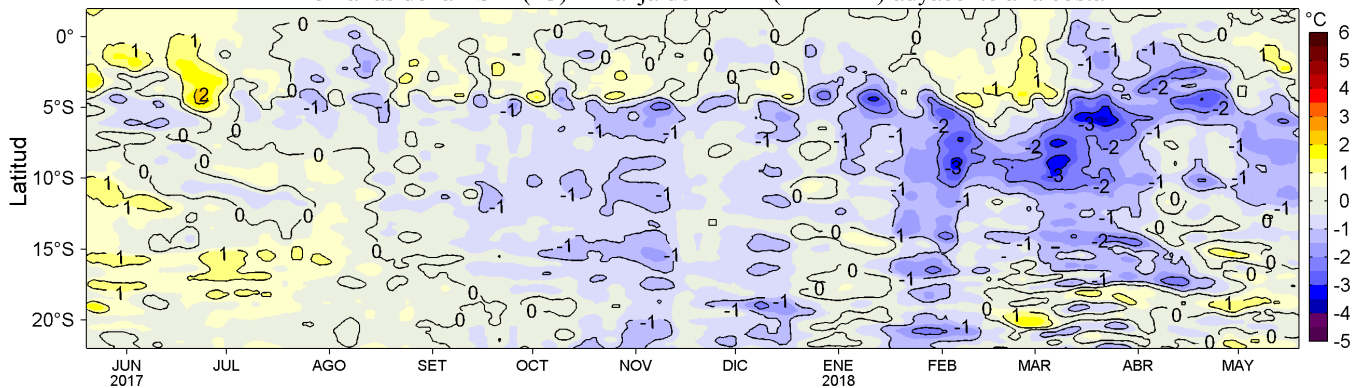
Figura 4. Variación promedio de las anomalías de la Temperatura Superficial del Mar (°C) para una franja de 60 mn (~111 km) adyacente al litoral peruano para los últimos doce meses al 19 de mayo de 2018. Datos: OSTIA-UKMO-L4-GLOB-v2.0 (UK Met. Office, 2012; Donlon et al, 2012) disponible en https://podaac.jpl.nasa.gov/dataset/OSTIA-UKMO-L4-GLOB-v2.0 . Las anomalías se calcularon con respecto al periodo 2007-2016. Procesamiento: LHF/AFIOF/DGIOCC/IMARPE.
