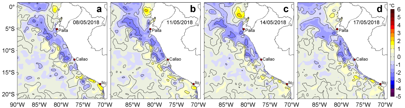
Figura 3. Anomalías de la Temperatura Superficial del Mar (°C) para los días: a) 08, b) 11, c) 14 y d) 17 de mayo de 2018. Las anomalías se calcularon respecto de la climatología para el periodo 2007-2016. Datos: OSTIA-UKMO-L4-GLOB-v2.0 (UK Met Office, 2012; Donlon et al, 2012). Procesamiento: LHF/AFIOF/DGIOCC/IMARPE.
