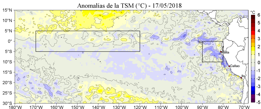
Figura 1. Anomalías de la Temperatura Superficial del Mar ( ^{\circ}\text{C} ) en el océano Pacífico tropical. Las regiones Niño 3.4 (5°N-5°S, 170°W-120°W) y Niño 1+2 (0°-10°S, 90°W-80°W) en los sectores central y oriental del océano, respectivamente, están delimitadas con una línea de color negro. Climatología: 2007-2016. Datos: OSTIA-UKMO-L4-GLOB-v2.0 (UK Met Office, 2012; Donlon et al, 2012) disponible en https://podaac.jpl.nasa.gov/dataset/OSTIA-UKMO-L4-GLOB-v2.0 . Procesamiento: LHFM/AFIOF/DGIOCC/IMARPE.
