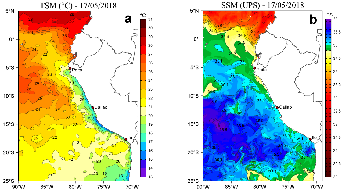
Figura 2. a) Temperatura Superficial del Mar (°C) y b) Salinidad Superficial del Mar (UPS) para el 17 de mayo de 2018. Datos: OSTIA-UKMO-L4-GLOB-v2.0 (UK Met Office, 2012; Donlon et al, 2012) disponible en https://podaac.jpl.nasa.gov/dataset/OSTIA-UKMO-L4-GLOB-v2.0 para (a) y Hybrid Coordinate Ocean Model (HYCOM; Halliwell et al., 1998; 2000; Bleck, 2001) para (b). Procesamiento: LHF/AFIOF/DGIOCC/IMARPE.
