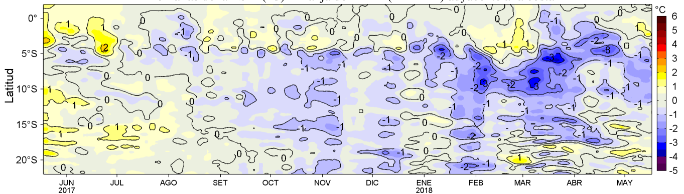
Figura 4. Variación promedio de las anomalías de la Temperatura Superficial del Mar (°C) para una franja de 60 mn (~111 km) adyacente al litoral peruano para los últimos doce meses al 17 de mayo de 2018. Datos: OSTIA-UKMO-L4-GLOB-v2.0 (UK Met. Office, 2012; Donlon et al, 2012) disponible en https://podaac.jpl.nasa.gov/dataset/OSTIA-UKMO-L4-GLOB-v2.0 . Las anomalías se calcularon con respecto al periodo 2007-2016. Procesamiento: LHF/AFIOF/DGIOCC/IMARPE.
