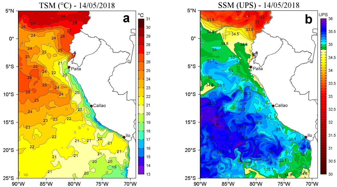
Figura 2. a) Temperatura Superficial del Mar ( ^{\circ}\text{C} ) y b) Salinidad Superficial del Mar (UPS) para el 14 de mayo de 2018. Datos: OSTIA-UKMO-L4-GLOB-v2.0 (UK Met Office, 2012; Donlon et al, 2012) disponible en https://podaac.jpl.nasa.gov/dataset/OSTIA-UKMO-L4-GLOB-v2.0 para (a) y Hybrid Coordinate Ocean Model (HYCOM; Halliwell et al., 1998; 2000; Bleck, 2001) para (b). Procesamiento: LHF/AFIOF/DGIOCC/IMARPE.
