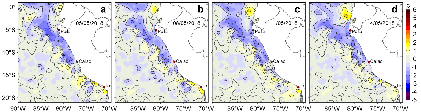
Figura 3. Anomalías de la Temperatura Superficial del Mar ( ^{\circ}\text{C} ) para los días: a) 05, b) 08, c) 11 y d) 14 de mayo de 2018. Las anomalías se calcularon respecto de la climatología para el periodo 2007-2016. Datos: OSTIA-UKMO-L4-GLOB-v2.0 (UK Met Office, 2012; Donlon et al, 2012). Procesamiento: LHF/AFIOF/DGIOCC/IMARPE.
