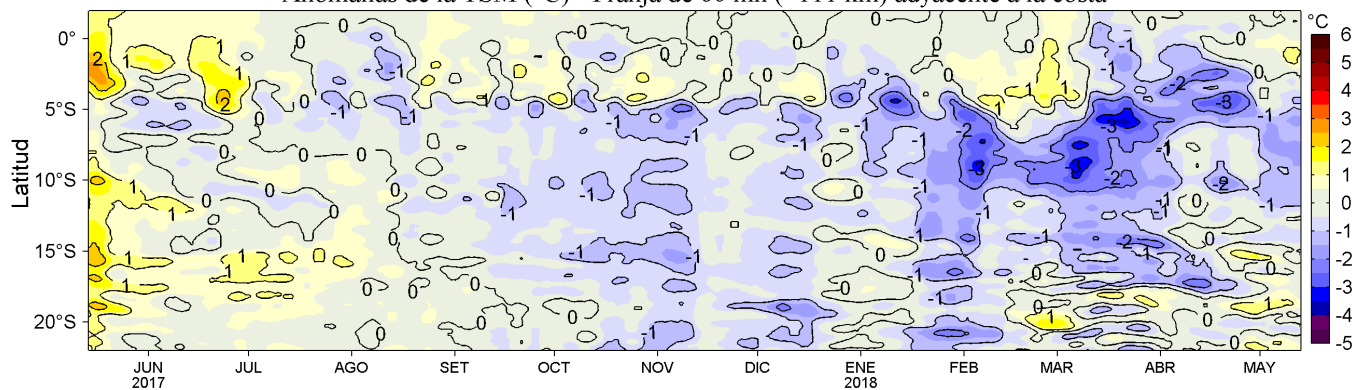
Figura 4. Variación promedio de las anomalías de la Temperatura Superficial del Mar (°C) para una franja de 60 mn (~111 km) adyacente al litoral peruano para los últimos doce meses al 13 de mayo de 2018. Datos: OSTIA-UKMO-L4-GLOB-v2.0 (UK Met. Office, 2012; Donlon et al, 2012) disponible en https://podaac.jpl.nasa.gov/dataset/OSTIA-UKMO-L4-GLOB-v2.0 . Las anomalías se calcularon con respecto al periodo 2007-2016. Procesamiento: LHF/AFIOF/DGIOCC/IMARPE.
