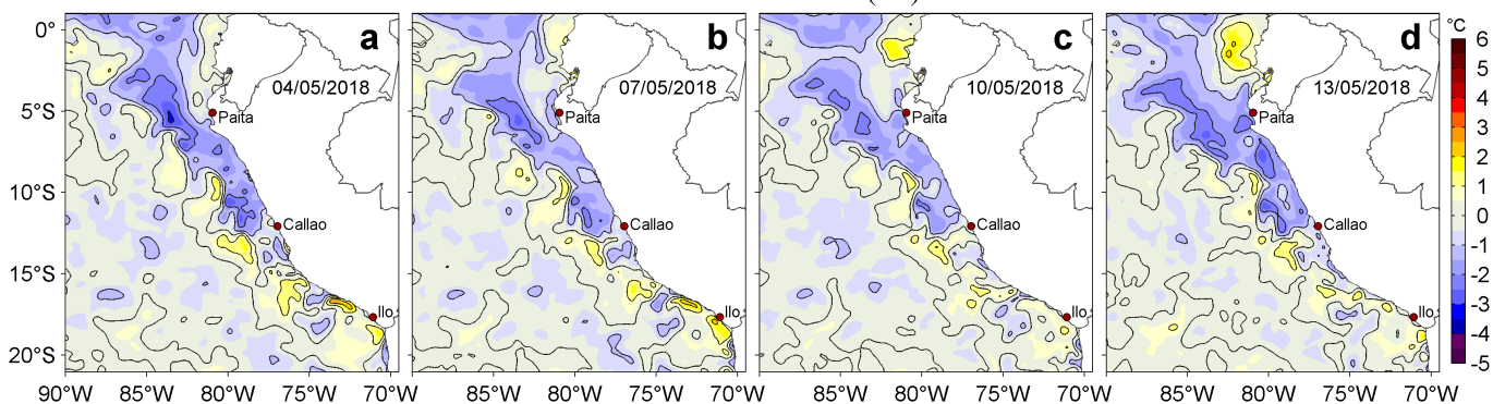
Figura 3. Anomalías de la Temperatura Superficial del Mar (°C) para los días: a) 04, b) 07, c) 10 y d) 13 de mayo de 2018. Las anomalías se calcularon respecto de la climatología para el periodo 2007-2016. Datos: OSTIA-UKMO-L4-GLOB-v2.0 (UK Met Office, 2012; Donlon et al, 2012). Procesamiento: LHF/AFIOF/DGIOCC/IMARPE.
