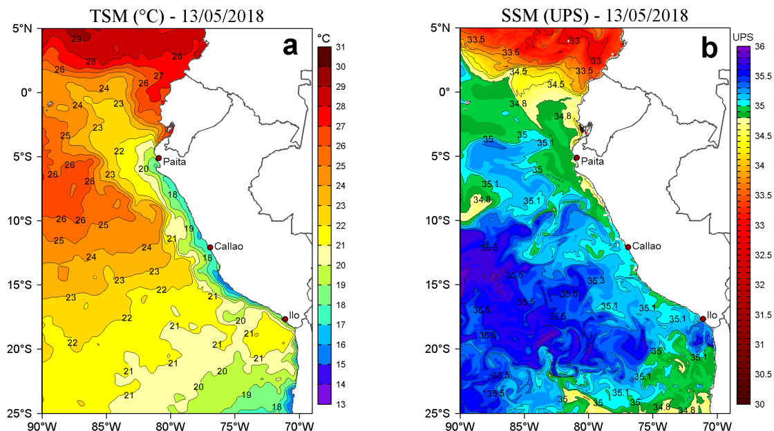
Figura 2. a) Temperatura Superficial del Mar (°C) y b) Salinidad Superficial del Mar (UPS) para el 13 de mayo de 2018. Datos: OSTIA-UKMO-L4-GLOB-v2.0 (UK Met Office, 2012; Donlon et al, 2012) disponible en https://podaac.jpl.nasa.gov/dataset/OSTIA-UKMO-L4-GLOB-v2.0 para (a) y Hybrid Coordinate Ocean Model (HYCOM; Halliwell et al., 1998; 2000; Bleck, 2001) para (b). Procesamiento: LHF/AFIOF/DGIOCC/IMARPE.
