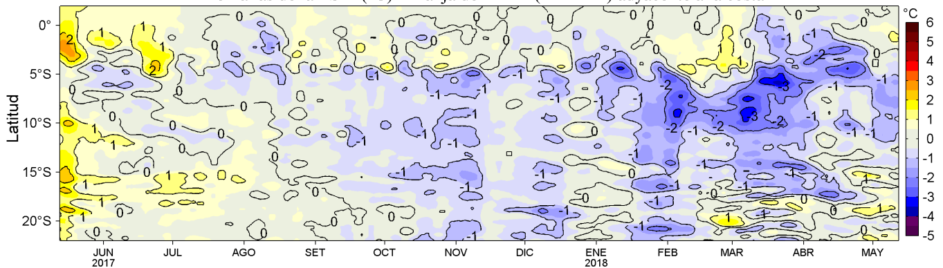
Figura 4. Variación promedio de las anomalías de la Temperatura Superficial del Mar (°C) para una franja de 60 mn (~111 km) adyacente al litoral peruano para los últimos doce meses al 12 de mayo de 2018. Datos: OSTIA-UKMO-L4-GLOB-v2.0 (UK Met. Office, 2012; Donlon et al, 2012) disponible en https://podaac.jpl.nasa.gov/dataset/OSTIA-UKMO-L4-GLOB-v2.0 . Las anomalías se calcularon con respecto al periodo 2007-2016. Procesamiento: LHF/AFIOF/DGIOCC/IMARPE.
