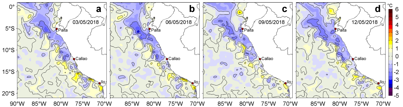
Figura 3. Anomalías de la Temperatura Superficial del Mar (°C) para los días: a) 03, b) 06, c) 09 y d) 12 de mayo de 2018. Las anomalías se calcularon respecto de la climatología para el periodo 2007-2016. Datos: OSTIA-UKMO-L4-GLOB-v2.0 (UK Met Office, 2012; Donlon et al, 2012). Procesamiento: LHF/AFIOF/DGIOCC/IMARPE.
