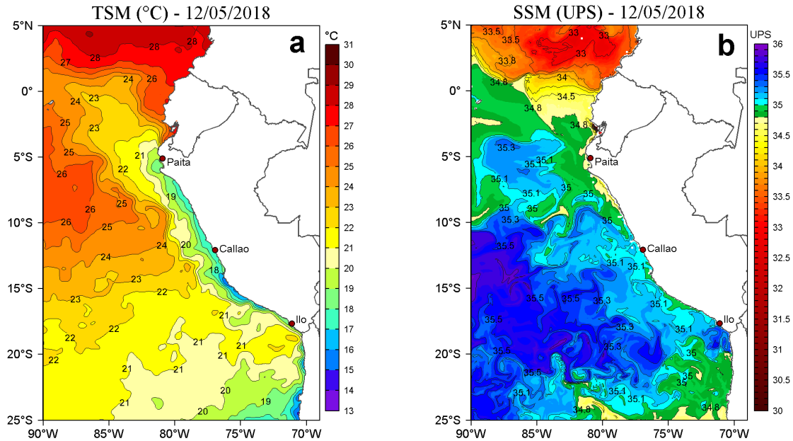
Figura 2. a) Temperatura Superficial del Mar (°C) y b) Salinidad Superficial del Mar (UPS) para el 12 de mayo de 2018. Datos: OSTIA-UKMO-L4-GLOB-v2.0 (UK Met Office, 2012; Donlon et al, 2012) disponible en https://podaac.jpl.nasa.gov/dataset/OSTIA-UKMO-L4-GLOB-v2.0 para (a) y Hybrid Coordinate Ocean Model (HYCOM; Halliwell et al., 1998; 2000; Bleck, 2001) para (b). Procesamiento: LHF/AFIOF/DGIOCC/IMARPE.
