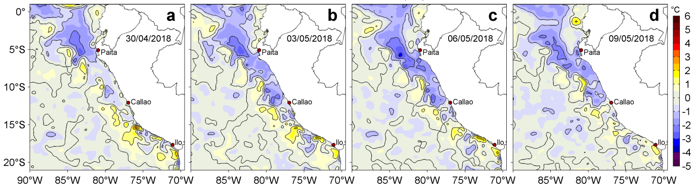
Figura 3. Anomalías de la Temperatura Superficial del Mar ( ^{\circ}\text{C} ) para los días: a) 30 de abril, b) 03, c) 06 y d) 09 de mayo de 2018. Las anomalías se calcularon respecto de la climatología para el periodo 2007-2016. Datos: OSTIA-UKMO-L4-GLOB-v2.0 (UK Met Office, 2012; Donlon et al, 2012). Procesamiento: LHF/AFIOF/DGIOCC/IMARPE.
