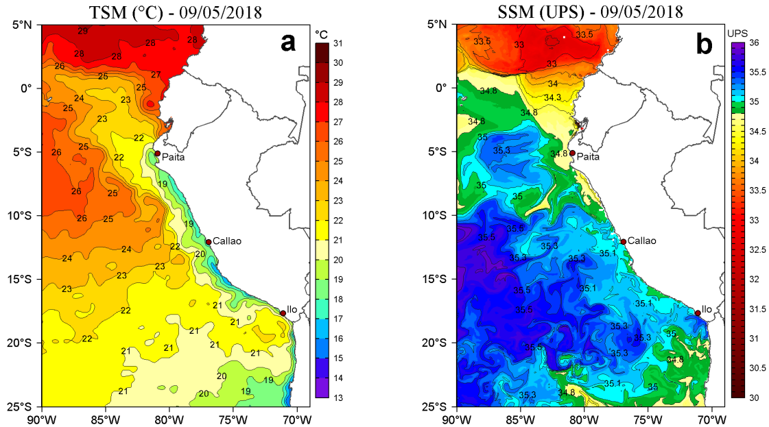
Figura 2. a) Temperatura Superficial del Mar ( ^{\circ}\text{C} ) y b) Salinidad Superficial del Mar (UPS) para el 09 de mayo de 2018. Datos: OSTIA-UKMO-L4-GLOB-v2.0 (UK Met Office, 2012; Donlon et al, 2012) disponible en https://podaac.jpl.nasa.gov/dataset/OSTIA-UKMO-L4-GLOB-v2.0 para (a) y Hybrid Coordinate Ocean Model (HYCOM; Halliwell et al., 1998; 2000; Bleck, 2001) para (b). Procesamiento: LHF/AFIOF/DGIOCC/IMARPE.
