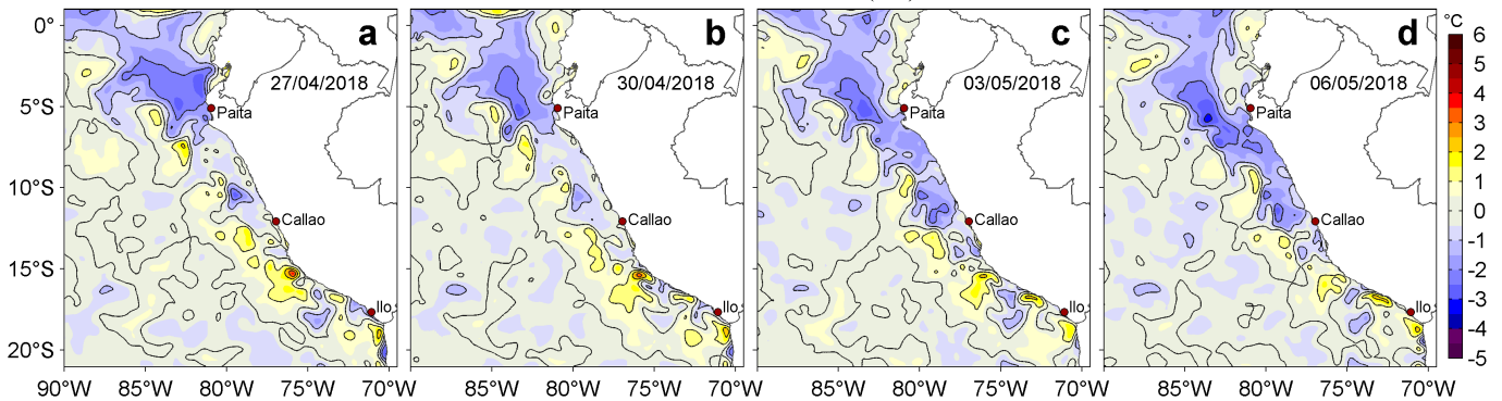
Figura 3. Anomalías de la Temperatura Superficial del Mar ( ^{\circ}\text{C} ) para los días: a) 27 y b) 30 de abril, c) 03 y d) 06 de mayo de 2018. Las anomalías se calcularon respecto de la climatología para el periodo 2007-2016. Datos: OSTIA-UKMO-L4-GLOB-v2.0 (UK Met Office, 2012; Donlon et al, 2012). Procesamiento: LHF/AFIOF/DGIOCC/IMARPE.
