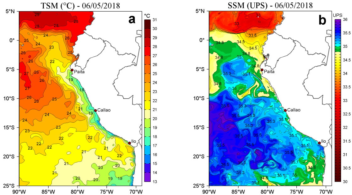
Figura 2. a) Temperatura Superficial del Mar ( ^{\circ}\text{C} ) y b) Salinidad Superficial del Mar (UPS) para el 06 de mayo de 2018. Datos: OSTIA-UKMO-L4-GLOB-v2.0 (UK Met Office, 2012; Donlon et al, 2012) disponible en https://podaac.jpl.nasa.gov/dataset/OSTIA-UKMO-L4-GLOB-v2.0 para (a) y Hybrid Coordinate Ocean Model (HYCOM; Halliwell et al., 1998; 2000; Bleck, 2001) para (b). Procesamiento: LHF/AFIOF/DGIOCC/IMARPE.
