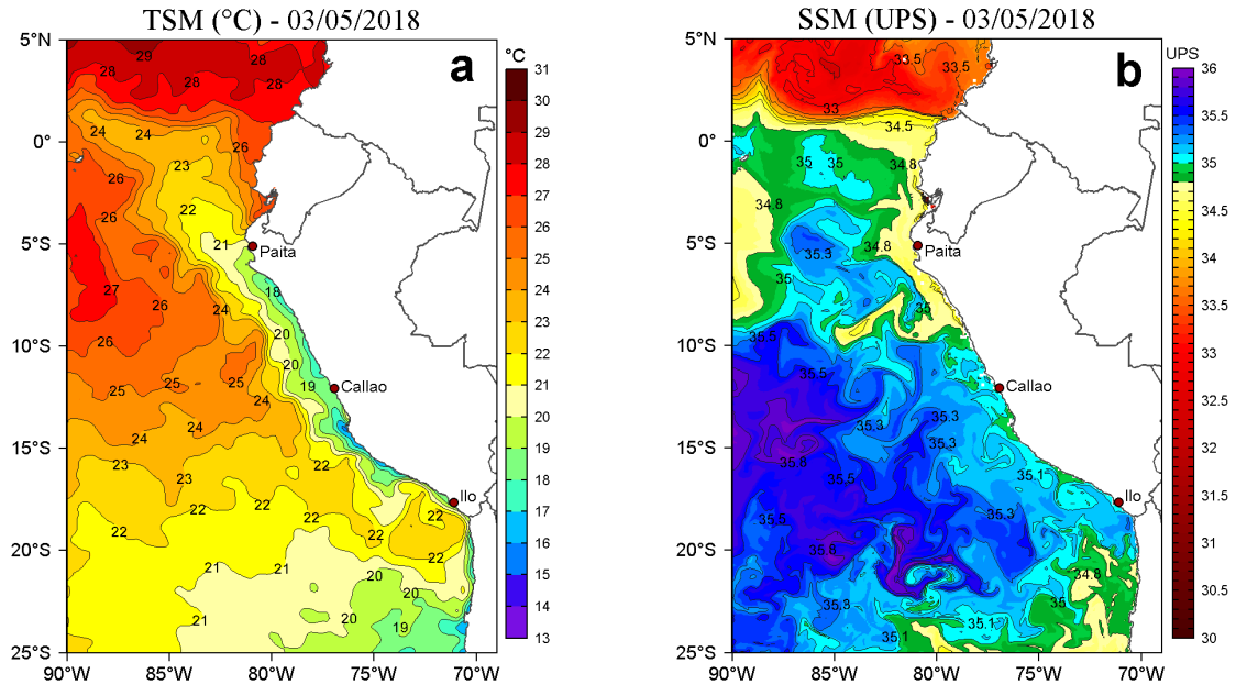
Figura 2. a) Temperatura Superficial del Mar ( ^{\circ}\text{C} ) y b) Salinidad Superficial del Mar (UPS) para el 03 de mayo de 2018. Datos: OSTIA-UKMO-L4-GLOB-v2.0 (UK Met Office, 2012; Donlon et al, 2012) disponible en https://podaac.jpl.nasa.gov/dataset/OSTIA-UKMO-L4-GLOB-v2.0 para (a) y Hybrid Coordinate Ocean Model (HYCOM; Halliwell et al., 1998; 2000; Bleck, 2001) para (b). Procesamiento: LHF/AFIOF/DGIOCC/IMARPE.
