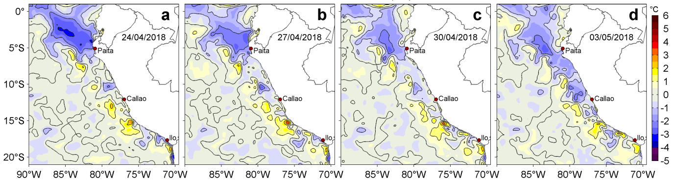
Figura 3. Anomalías de la Temperatura Superficial del Mar ( ^{\circ}\text{C} ) para los días: a) 24, b) 27, c) 30 de abril y d) 03 de mayo de 2018. Las anomalías se calcularon respecto de la climatología para el periodo 2007-2016. Datos: OSTIA-UKMO-L4-GLOB-v2.0 (UK Met Office, 2012; Donlon et al, 2012). Procesamiento: LHF/AFIOF/DGIOCC/IMARPE.
