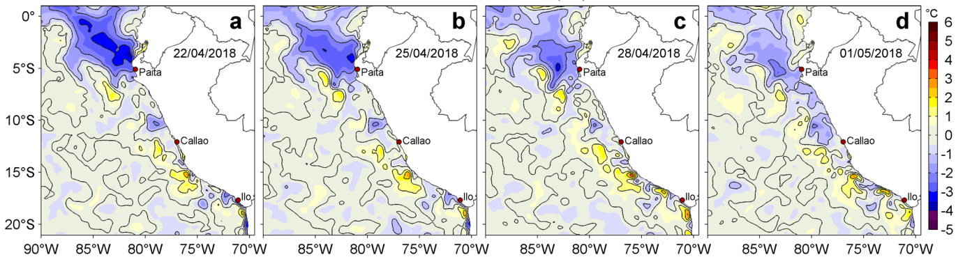
Figura 3. Anomalías de la Temperatura Superficial del Mar ( ^{\circ}\text{C} ) para los días: a) 22, b) 25, c) 28 de abril y d) 01 de mayo de 2018. Las anomalías se calcularon respecto de la climatología para el periodo 2007-2016. Datos: OSTIA-UKMO-L4-GLOB-v2.0 (UK Met Office, 2012; Donlon et al, 2012). Procesamiento: LHFM/AFIOF/DGIOCC/IMARPE.
