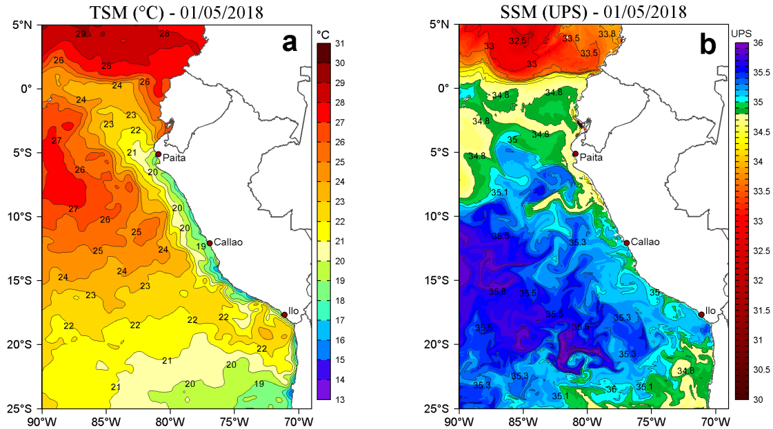
Figura 2. a) Temperatura Superficial del Mar ( ^{\circ}\text{C} ) y b) Salinidad Superficial del Mar (UPS) para el 01 de mayo de 2018. Datos: OSTIA-UKMO-L4-GLOB-v2.0 (UK Met Office, 2012; Donlon et al, 2012) disponible en https://podaac.jpl.nasa.gov/dataset/OSTIA-UKMO-L4-GLOB-v2.0 para (a) y Hybrid Coordinate Ocean Model (HYCOM; Halliwell et al., 1998; 2000; Bleck, 2001) para (b). Procesamiento: LHFM/AFIOF/DGIOCC/IMARPE.
