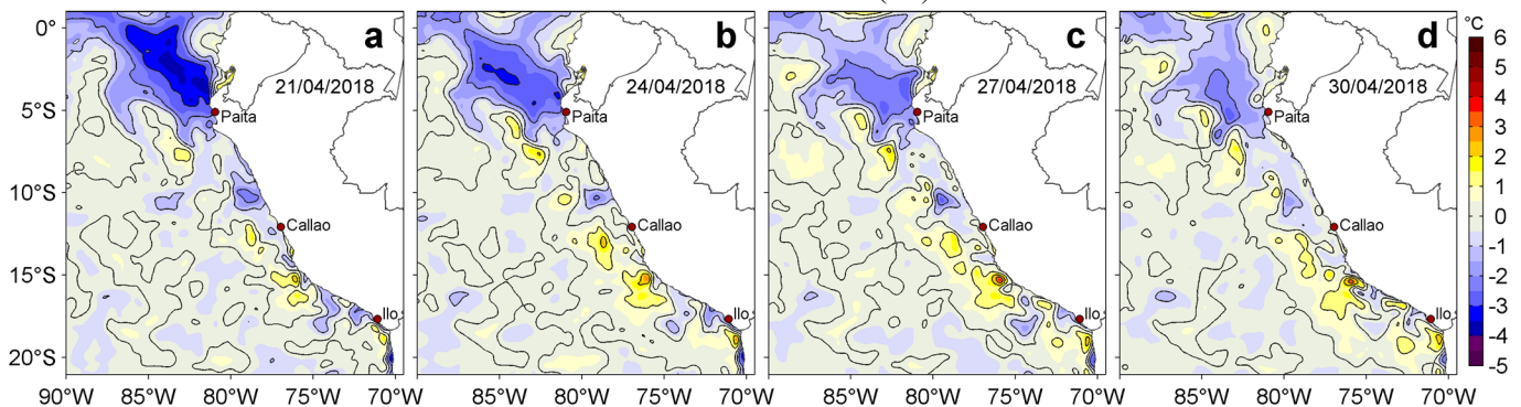
Figura 3. Anomalías de la Temperatura Superficial del Mar ( ^{\circ}\text{C} ) para los días: a) 21, b) 24, c) 27 y d) 30 de abril de 2018. Las anomalías se calcularon respecto de la climatología para el periodo 2007-2016. Datos: OSTIA-UKMO-L4-GLOB-v2.0 (UK Met Office, 2012; Donlon et al, 2012). Procesamiento: LHF/AFIOF/DGIOCC/IMARPE.
