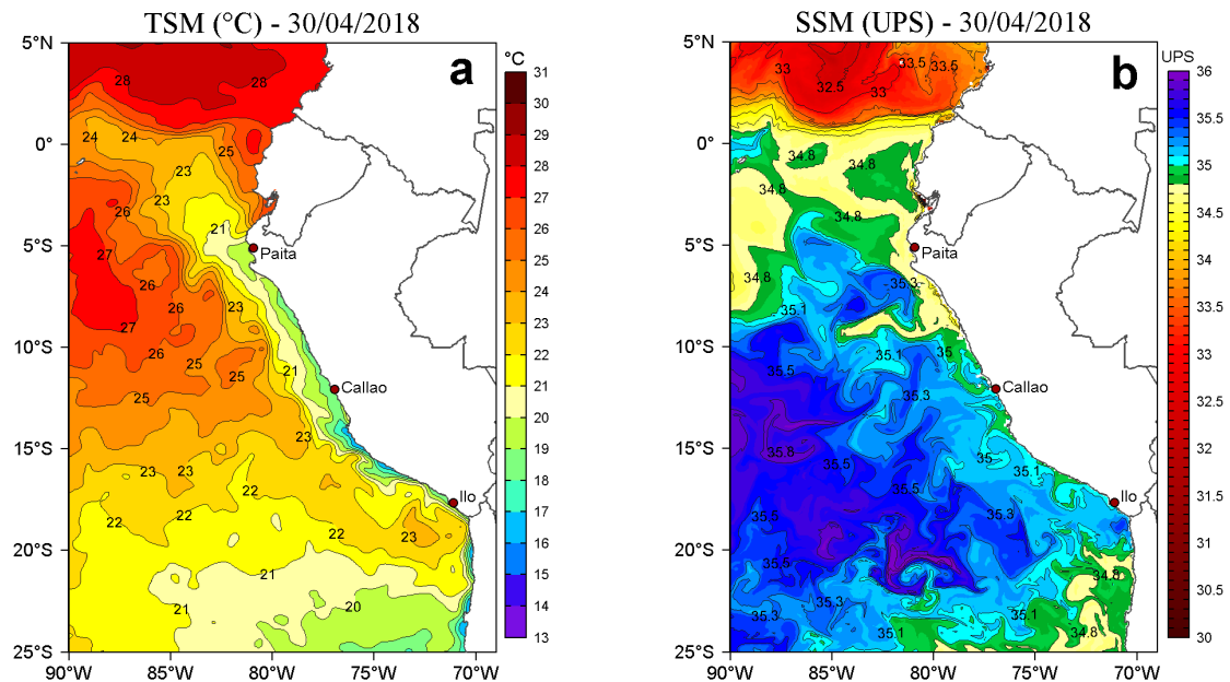
Figura 2. a) Temperatura Superficial del Mar ( ^{\circ}\text{C} ) y b) Salinidad Superficial del Mar (UPS) para el 30 de abril de 2018. Datos: OSTIA-UKMO-L4-GLOB-v2.0 (UK Met Office, 2012; Donlon et al, 2012) disponible en https://podaac.jpl.nasa.gov/dataset/OSTIA-UKMO-L4-GLOB-v2.0 para (a) y Hybrid Coordinate Ocean Model (HYCOM; Halliwell et al., 1998; 2000; Bleck, 2001) para (b). Procesamiento: LHF/AFIOF/DGIOCC/IMARPE.
