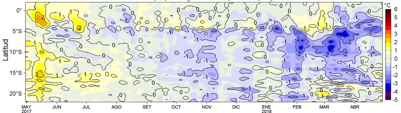
Figura 4. Variación promedio de las anomalías de la Temperatura Superficial del Mar (°C) para una franja de 60 mn (~111 km) adyacente al litoral peruano para los últimos doce meses al 29 de abril de 2018. Datos: OSTIA-UKMO-L4-GLOB-v2.0 (UK Met. Office, 2012; Donlon et al, 2012) disponible en https://podaac.jpl.nasa.gov/dataset/OSTIA-UKMO-L4-GLOB-v2.0 . Las anomalías se calcularon con respecto al periodo 2007-2016. Procesamiento: LHF/AFIOF/DGIOCC/IMARPE.
