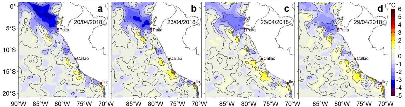
Figura 3. Anomalías de la Temperatura Superficial del Mar (°C) para los días: a) 20, b) 23, c) 26 y d) 29 de abril de 2018. Las anomalías se calcularon respecto de la climatología para el periodo 2007-2016. Datos: OSTIA-UKMO-L4-GLOB-v2.0 (UK Met Office, 2012; Donlon et al, 2012). Procesamiento: LHF/AFIOF/DGIOCC/IMARPE.
