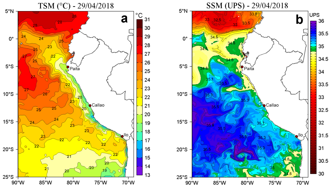
Figura 2. a) Temperatura Superficial del Mar (°C) y b) Salinidad Superficial del Mar (UPS) para el 29 de abril de 2018. Datos: OSTIA-UKMO-L4-GLOB-v2.0 (UK Met Office, 2012; Donlon et al, 2012) disponible en https://podaac.jpl.nasa.gov/dataset/OSTIA-UKMO-L4-GLOB-v2.0 para (a) y Hybrid Coordinate Ocean Model (HYCOM; Halliwell et al., 1998; 2000; Bleck, 2001) para (b). Procesamiento: LHF/AFIOF/DGIOCC/IMARPE.
