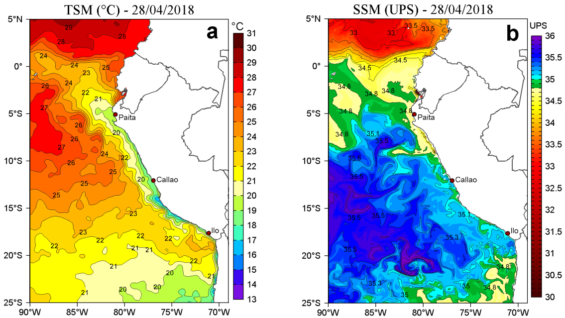
Figura 2. a) Temperatura Superficial del Mar (°C) y b) Salinidad Superficial del Mar (UPS) para el 28 de abril de 2018. Datos: OSTIA-UKMO-L4-GLOB-v2.0 (UK Met Office, 2012; Donlon et al, 2012) disponible en https://podaac.jpl.nasa.gov/dataset/OSTIA-UKMO-L4-GLOB-v2.0 para (a) y Hybrid Coordinate Ocean Model (HYCOM; Halliwell et al., 1998; 2000; Bleck, 2001) para (b). Procesamiento: LHF/AFIOF/DGIOCC/IMARPE.
