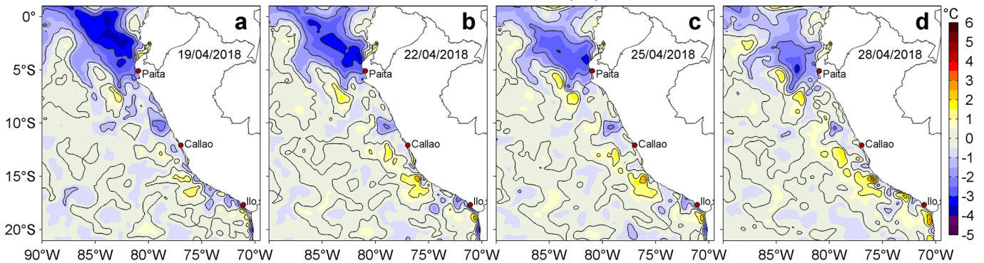
Figura 3. Anomalías de la Temperatura Superficial del Mar (°C) para los días: a) 19, b) 22, c) 25 y d) 28 de abril de 2018. Las anomalías se calcularon respecto de la climatología para el periodo 2007-2016. Datos: OSTIA-UKMO-L4-GLOB-v2.0 (UK Met Office, 2012; Donlon et al, 2012). Procesamiento: LHF/AFIOF/DGIOCC/IMARPE.
