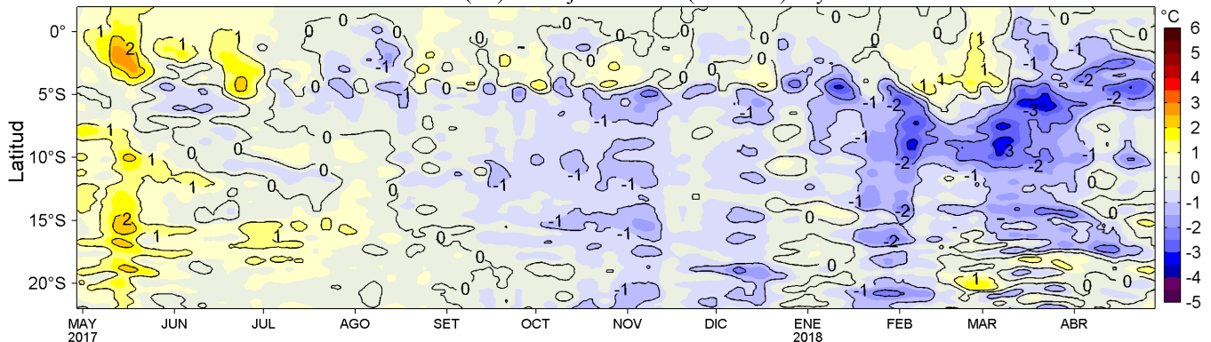
Figura 4. Variación promedio de las anomalías de la Temperatura Superficial del Mar (°C) para una franja de 60 mn (~111 km) adyacente al litoral peruano para los últimos doce meses al 28 de abril de 2018. Datos: OSTIA-UKMO-L4-GLOB-v2.0 (UK Met. Office, 2012; Donlon et al, 2012) disponible en https://podaac.jpl.nasa.gov/dataset/OSTIA-UKMO-L4-GLOB-v2.0 . Las anomalías se calcularon con respecto al periodo 2007-2016. Procesamiento: LHF/AFIOF/DGIOCC/IMARPE.
