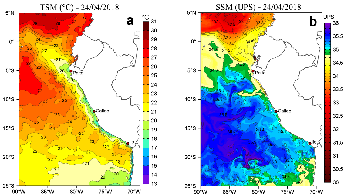
Figura 2. a) Temperatura Superficial del Mar ( ^{\circ}\text{C} ) y b) Salinidad Superficial del Mar (UPS) para el 24 de abril de 2018. Datos: OSTIA-UKMO-L4-GLOB-v2.0 (UK Met Office, 2012; Donlon et al, 2012) disponible en https://podaac.jpl.nasa.gov/dataset/OSTIA-UKMO-L4-GLOB-v2.0 para (a) y Hybrid Coordinate Ocean Model (HYCOM; Halliwell et al., 1998; 2000; Bleck, 2001) para (b). Procesamiento: LHF/AFIOF/DGIOCC/IMARPE.
