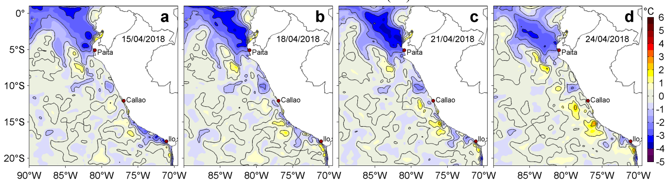
Figura 3. Anomalías de la Temperatura Superficial del Mar ( ^{\circ}\text{C} ) para los días: a) 15, b) 18, c) 21 y d) 24 de abril de 2018. Las anomalías se calcularon respecto de la climatología para el periodo 2007-2016. Datos: OSTIA-UKMO-L4-GLOB-v2.0 (UK Met Office, 2012; Donlon et al, 2012). Procesamiento: LHF/AFIOF/DGIOCC/IMARPE.
