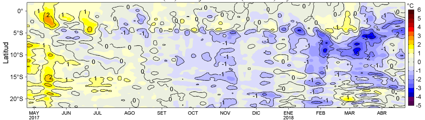
Figura 4. Variación promedio de las anomalías de la Temperatura Superficial del Mar (°C) para una franja de 60 mn (~111 km) adyacente al litoral peruano para los últimos doce meses al 23 de abril de 2018. Datos: OSTIA-UKMO-L4-GLOB-v2.0 (UK Met. Office, 2012; Donlon et al, 2012) disponible en https://podaac.jpl.nasa.gov/dataset/OSTIA-UKMO-L4-GLOB-v2.0 . Las anomalías se calcularon con respecto al periodo 2007-2016. Procesamiento: LHFM/AFIOF/DGIOCC/IMARPE.
