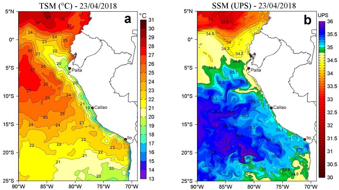
Figura 2. a) Temperatura Superficial del Mar (°C) y b) Salinidad Superficial del Mar (UPS) para el 23 de abril de 2018. Datos: OSTIA-UKMO-L4-GLOB-v2.0 (UK Met Office, 2012; Donlon et al, 2012) disponible en https://podaac.jpl.nasa.gov/dataset/OSTIA-UKMO-L4-GLOB-v2.0 para (a) y Hybrid Coordinate Ocean Model (HYCOM; Halliwell et al., 1998; 2000; Bleck, 2001) para (b). Procesamiento: LHFM/AFIOF/DGIOCC/IMARPE.
