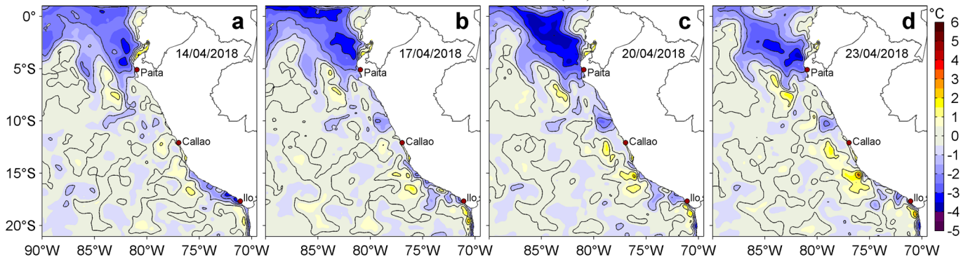
Figura 3. Anomalías de la Temperatura Superficial del Mar (°C) para los días: a) 14, b) 17, c) 20 y d) 23 de abril de 2018. Las anomalías se calcularon respecto de la climatología para el periodo 2007-2016. Datos: OSTIA-UKMO-L4-GLOB-v2.0 (UK Met Office, 2012; Donlon et al, 2012). Procesamiento: LHFM/AFIOF/DGIOCC/IMARPE.
