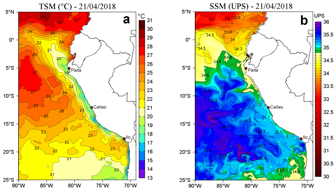
Figura 2. a) Temperatura Superficial del Mar ( ^{\circ}\text{C} ) y b) Salinidad Superficial del Mar (UPS) para el 21 de abril de 2018. Datos: OSTIA-UKMO-L4-GLOB-v2.0 (UK Met Office, 2012; Donlon et al, 2012) disponible en https://podaac.jpl.nasa.gov/dataset/OSTIA-UKMO-L4-GLOB-v2.0 para (a) y Hybrid Coordinate Ocean Model (HYCOM; Halliwell et al., 1998; 2000; Bleck, 2001) para (b). Procesamiento: LHF/AFIOF/DGIOCC/IMARPE.
