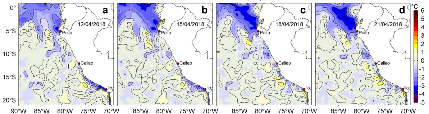
Figura 3. Anomalías de la Temperatura Superficial del Mar ( ^{\circ}\text{C} ) para los días: a) 12, b) 15, c) 18 y d) 21 de abril de 2018. Las anomalías se calcularon respecto de la climatología para el periodo 2007-2016. Datos: OSTIA-UKMO-L4-GLOB-v2.0 (UK Met Office, 2012; Donlon et al, 2012). Procesamiento: LHF/AFIOF/DGIOCC/IMARPE.
