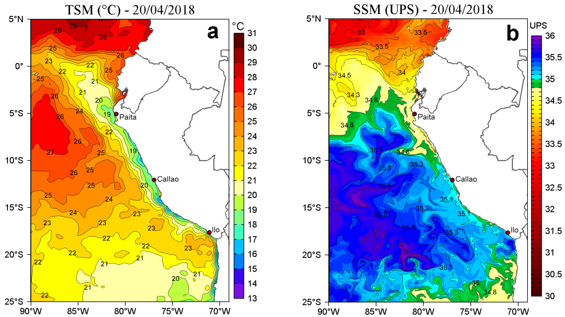
Figura 2. a) Temperatura Superficial del Mar ( ^{\circ}\text{C} ) y b) Salinidad Superficial del Mar (UPS) para el 20 de abril de 2018. Datos: OSTIA-UKMO-L4-GLOB-v2.0 (UK Met Office, 2012; Donlon et al, 2012) disponible en https://podaac.jpl.nasa.gov/dataset/OSTIA-UKMO-L4-GLOB-v2.0 para (a) y Hybrid Coordinate Ocean Model (HYCOM; Halliwell et al., 1998; 2000; Bleck, 2001) para (b). Procesamiento: LHF/AFIOF/DGIOCC/IMARPE.
