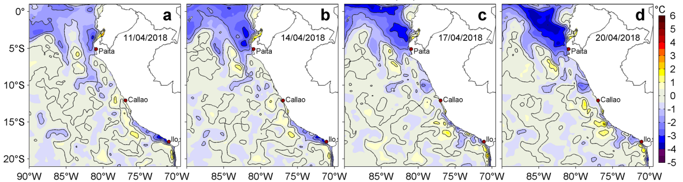
Figura 3. Anomalías de la Temperatura Superficial del Mar ( ^{\circ}\text{C} ) para los días: a) 11, b) 14, c) 17 y d) 20 de abril de 2018. Las anomalías se calcularon respecto de la climatología para el periodo 2007-2016. Datos: OSTIA-UKMO-L4-GLOB-v2.0 (UK Met Office, 2012; Donlon et al, 2012). Procesamiento: LHF/AFIOF/DGIOCC/IMARPE.
