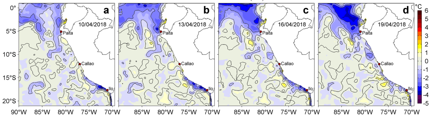
Figura 3. Anomalías de la Temperatura Superficial del Mar ( ^{\circ}\text{C} ) para los días: a) 10, b) 13, c) 16 y d) 19 de abril de 2018. Las anomalías se calcularon respecto de la climatología para el periodo 2007-2016. Datos: OSTIA-UKMO-L4-GLOB-v2.0 (UK Met Office, 2012; Donlon et al, 2012). Procesamiento: LHF/AFIOF/DGIOCC/IMARPE.
