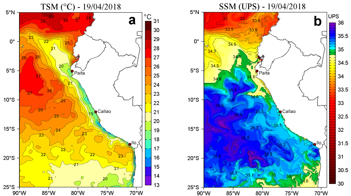
Figura 2. a) Temperatura Superficial del Mar ( ^{\circ}\text{C} ) y b) Salinidad Superficial del Mar (UPS) para el 19 de abril de 2018. Datos: OSTIA-UKMO-L4-GLOB-v2.0 (UK Met Office, 2012; Donlon et al, 2012) disponible en https://podaac.jpl.nasa.gov/dataset/OSTIA-UKMO-L4-GLOB-v2.0 para (a) y Hybrid Coordinate Ocean Model (HYCOM; Halliwell et al., 1998; 2000; Bleck, 2001) para (b). Procesamiento: LHF/AFIOF/DGIOCC/IMARPE.
