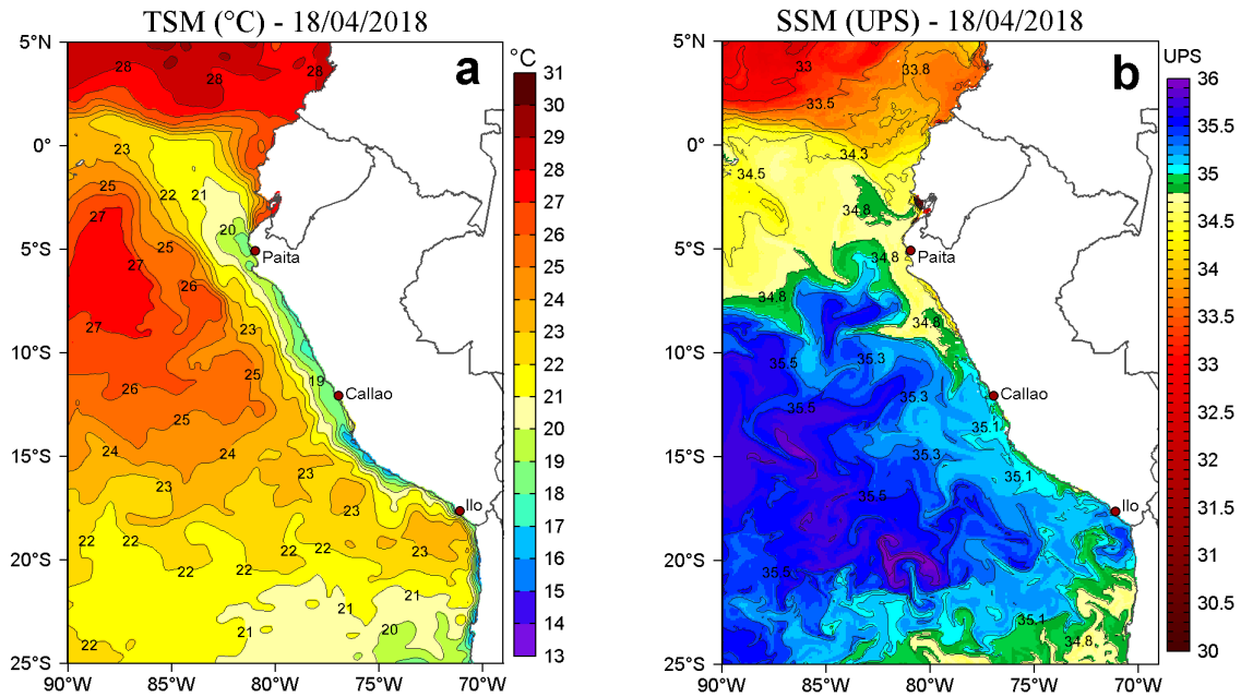
Figura 2. a) Temperatura Superficial del Mar ( ^{\circ}\text{C} ) y b) Salinidad Superficial del Mar (UPS) para el 18 de abril de 2018. Datos: OSTIA-UKMO-L4-GLOB-v2.0 (UK Met Office, 2012; Donlon et al, 2012) disponible en https://podaac.jpl.nasa.gov/dataset/OSTIA-UKMO-L4-GLOB-v2.0 para (a) y Hybrid Coordinate Ocean Model (HYCOM; Halliwell et al., 1998; 2000; Bleck, 2001) para (b). Procesamiento: LHF/AFIOF/DGIOCC/IMARPE.
