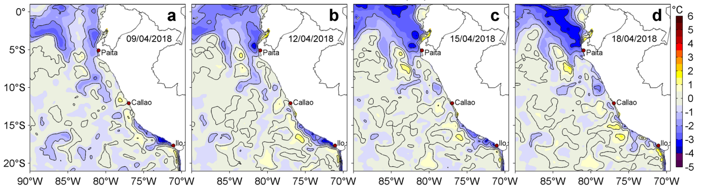
Figura 3. Anomalías de la Temperatura Superficial del Mar ( ^{\circ}\text{C} ) para los días: a) 09, b) 12, c) 15 y d) 18 de abril de 2018. Las anomalías se calcularon respecto de la climatología para el periodo 2007-2016. Datos: OSTIA-UKMO-L4-GLOB-v2.0 (UK Met Office, 2012; Donlon et al, 2012). Procesamiento: LHF/AFIOF/DGIOCC/IMARPE.
