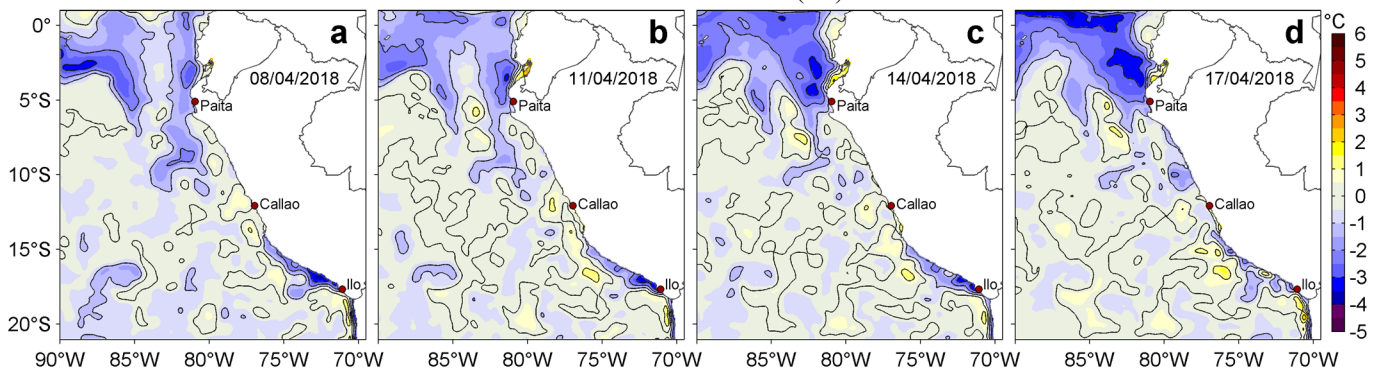
Figura 3. Anomalías de la Temperatura Superficial del Mar (°C) para los días: a) 08, b) 11, c) 14 y d) 17 de abril de 2018. Las anomalías se calcularon respecto de la climatología para el periodo 2007-2016. Datos: OSTIA-UKMO-L4-GLOB-v2.0 (UK Met Office, 2012; Donlon et al, 2012). Procesamiento: LHF/AFIOF/DGIOCC/IMARPE.
