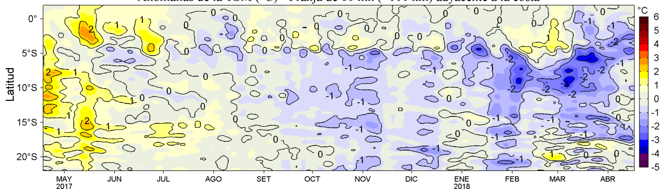
Figura 4. Variación promedio de las anomalías de la Temperatura Superficial del Mar (°C) para una franja de 60 mn (~111 km) adyacente al litoral peruano para los últimos doce meses al 17 de abril de 2018. Datos: OSTIA-UKMO-L4-GLOB-v2.0 (UK Met. Office, 2012; Donlon et al, 2012) disponible en https://podaac.jpl.nasa.gov/dataset/OSTIA-UKMO-L4-GLOB-v2.0 . Las anomalías se calcularon con respecto al periodo 2007-2016. Procesamiento: LHF/AFIOF/DGIOCC/IMARPE.
