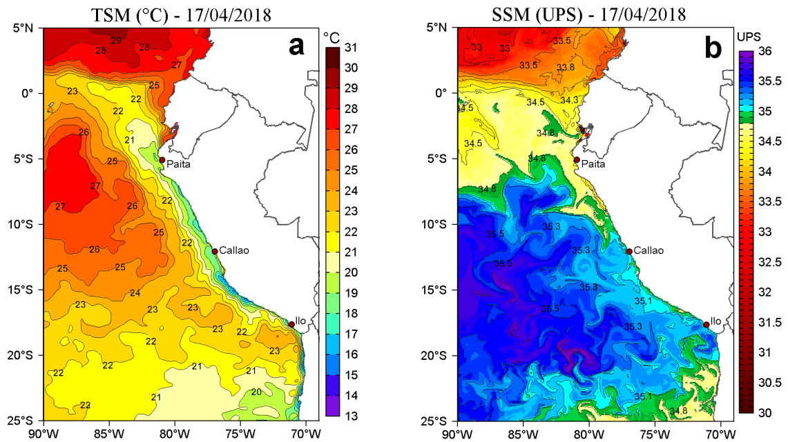
Figura 2. a) Temperatura Superficial del Mar (°C) y b) Salinidad Superficial del Mar (UPS) para el 17 de abril de 2018. Datos: OSTIA-UKMO-L4-GLOB-v2.0 (UK Met Office, 2012; Donlon et al, 2012) disponible en https://podaac.jpl.nasa.gov/dataset/OSTIA-UKMO-L4-GLOB-v2.0 para (a) y Hybrid Coordinate Ocean Model (HYCOM; Halliwell et al., 1998; 2000; Bleck, 2001) para (b). Procesamiento: LHF/AFIOF/DGIOCC/IMARPE.
