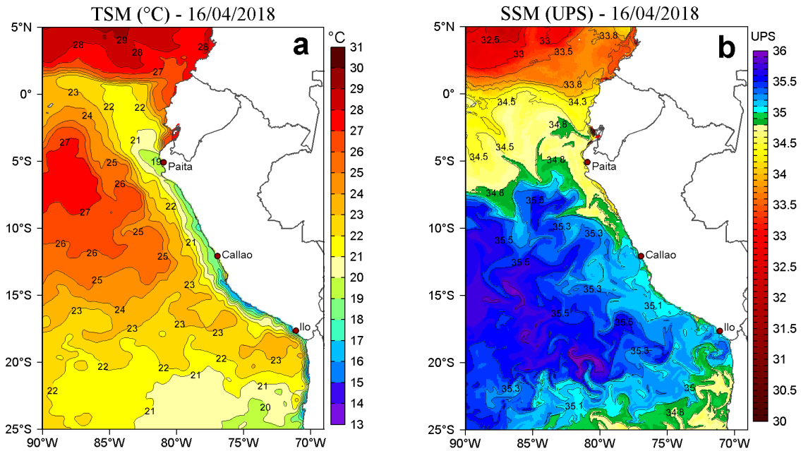
Figura 2. a) Temperatura Superficial del Mar ( ^{\circ}\text{C} ) y b) Salinidad Superficial del Mar (UPS) para el 16 de abril de 2018. Datos: OSTIA-UKMO-L4-GLOB-v2.0 (UK Met Office, 2012; Donlon et al, 2012) disponible en https://podaac.jpl.nasa.gov/dataset/OSTIA-UKMO-L4-GLOB-v2.0 para (a) y Hybrid Coordinate Ocean Model (HYCOM; Halliwell et al., 1998; 2000; Bleck, 2001) para (b). Procesamiento: LHF/AFIOF/DGIOCC/IMARPE.
