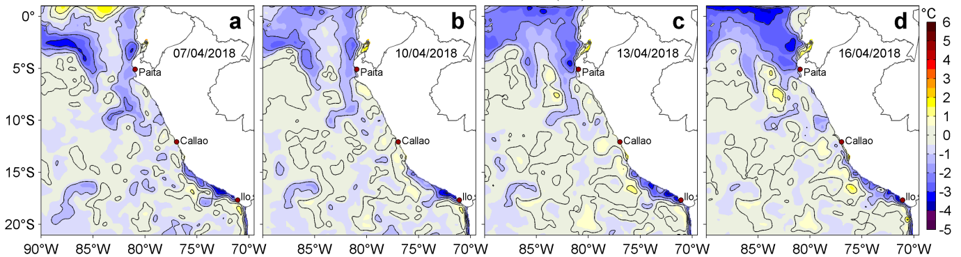
Figura 3. Anomalías de la Temperatura Superficial del Mar ( ^{\circ}\text{C} ) para los días: a) 07, b) 10, c) 13 y d) 16 de abril de 2018. Las anomalías se calcularon respecto de la climatología para el periodo 2007-2016. Datos: OSTIA-UKMO-L4-GLOB-v2.0 (UK Met Office, 2012; Donlon et al, 2012). Procesamiento: LHF/AFIOF/DGIOCC/IMARPE.
