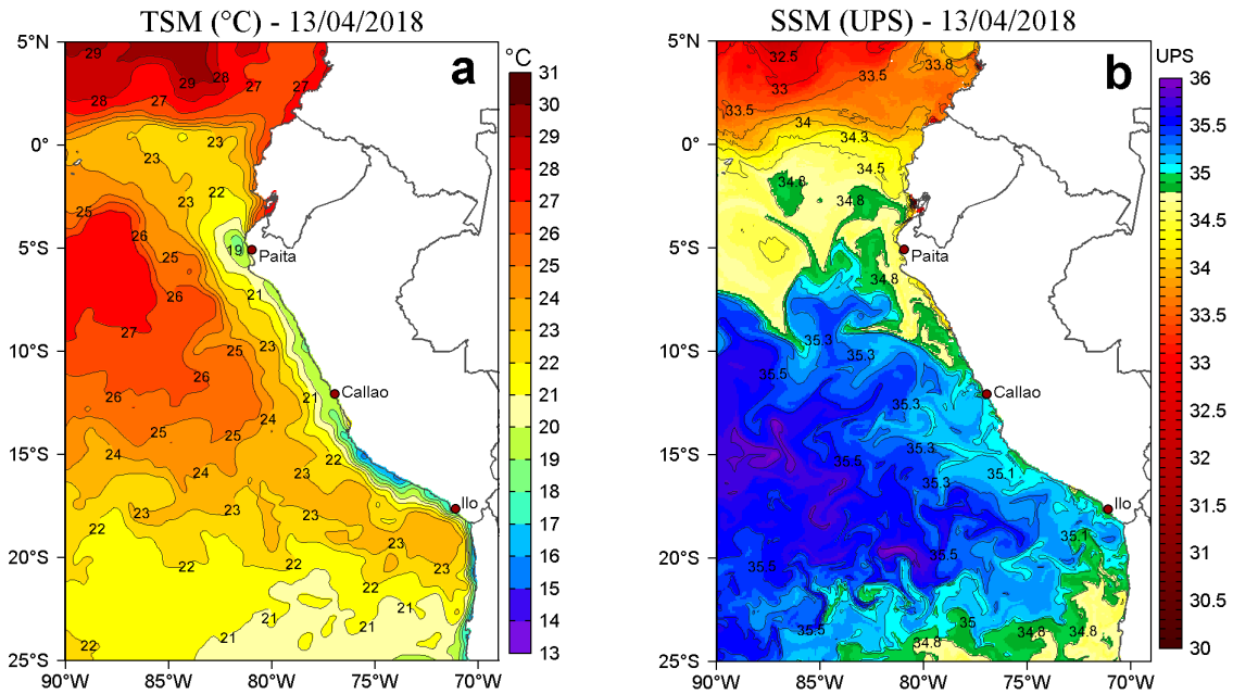
Figura 2. a) Temperatura Superficial del Mar ( ^{\circ}\text{C} ) y b) Salinidad Superficial del Mar (UPS) para el 13 de abril de 2018. Datos: OSTIA-UKMO-L4-GLOB-v2.0 (UK Met Office, 2012; Donlon et al, 2012) disponible en https://podaac.jpl.nasa.gov/dataset/OSTIA-UKMO-L4-GLOB-v2.0 para (a) y Hybrid Coordinate Ocean Model (HYCOM; Halliwell et al., 1998; 2000; Bleck, 2001) para (b). Procesamiento: LHF/AFIOF/DGIOCC/IMARPE.
