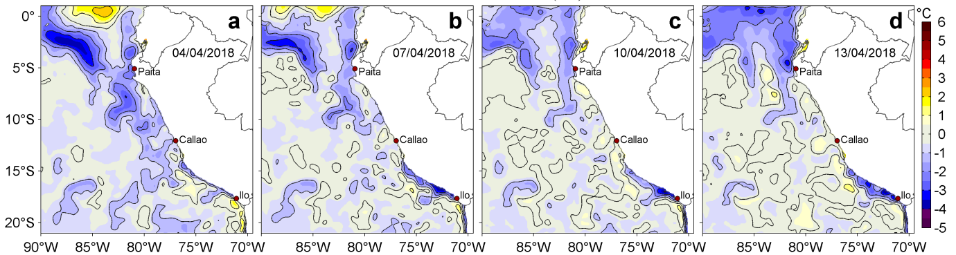
Figura 3. Anomalías de la Temperatura Superficial del Mar ( ^{\circ}\text{C} ) para los días: a) 04, b) 07, c) 10 y d) 13 de abril de 2018. Las anomalías se calcularon respecto de la climatología para el periodo 2007-2016. Datos: OSTIA-UKMO-L4-GLOB-v2.0 (UK Met Office, 2012; Donlon et al, 2012). Procesamiento: LHF/AFIOF/DGIOCC/IMARPE.
