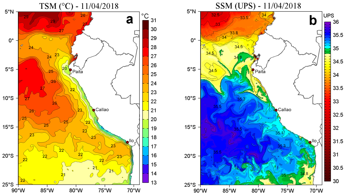
Figura 2. a) Temperatura Superficial del Mar (°C) y b) Salinidad Superficial del Mar (UPS) para el 11 de abril de 2018. Datos: OSTIA-UKMO-L4-GLOB-v2.0 (UK Met Office, 2012; Donlon et al, 2012) disponible en https://podaac.jpl.nasa.gov/dataset/OSTIA-UKMO-L4-GLOB-v2.0 para (a) y Hybrid Coordinate Ocean Model (HYCOM; Halliwell et al., 1998; 2000; Bleck, 2001) para (b). Procesamiento: LHF/AFIOF/DGIOCC/IMARPE.
