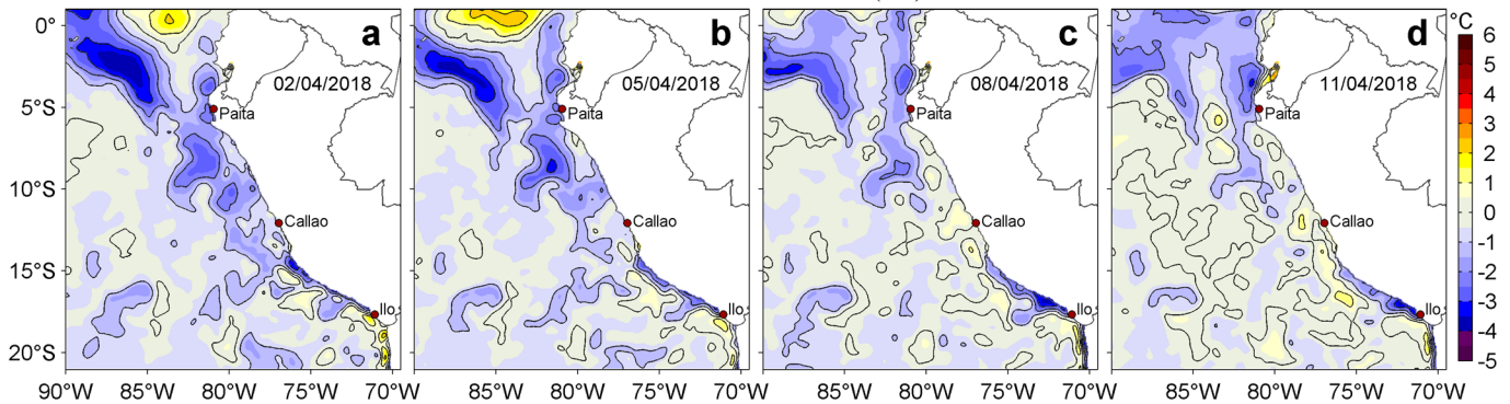
Figura 3. Anomalías de la Temperatura Superficial del Mar (°C) para los días: a) 02, b) 05, c) 08 y d) 11 de abril de 2018. Las anomalías se calcularon respecto de la climatología para el periodo 2007-2016. Datos: OSTIA-UKMO-L4-GLOB-v2.0 (UK Met Office, 2012; Donlon et al, 2012). Procesamiento: LHF/AFIOF/DGIOCC/IMARPE.
