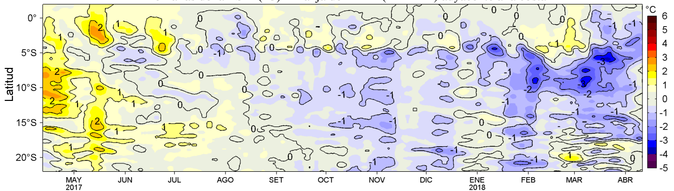
Figura 4. Variación promedio de las anomalías de la Temperatura Superficial del Mar (°C) para una franja de 60 mn (~111 km) adyacente al litoral peruano para los últimos doce meses al 11 de abril de 2018. Datos: OSTIA-UKMO-L4-GLOB-v2.0 (UK Met. Office, 2012; Donlon et al, 2012) disponible en https://podaac.jpl.nasa.gov/dataset/OSTIA-UKMO-L4-GLOB-v2.0 . Las anomalías se calcularon con respecto al periodo 2007-2016. Procesamiento: LHF/AFIOF/DGIOCC/IMARPE.
