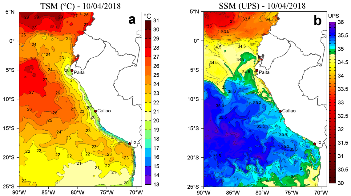
Figura 2. a) Temperatura Superficial del Mar ( ^{\circ}\text{C} ) y b) Salinidad Superficial del Mar (UPS) para el 10 de abril de 2018. Datos: OSTIA-UKMO-L4-GLOB-v2.0 (UK Met Office, 2012; Donlon et al, 2012) disponible en https://podaac.jpl.nasa.gov/dataset/OSTIA-UKMO-L4-GLOB-v2.0 para (a) y Hybrid Coordinate Ocean Model (HYCOM; Halliwell et al., 1998; 2000; Bleck, 2001) para (b). Procesamiento: LHF/AFIOF/DGIOCC/IMARPE.
