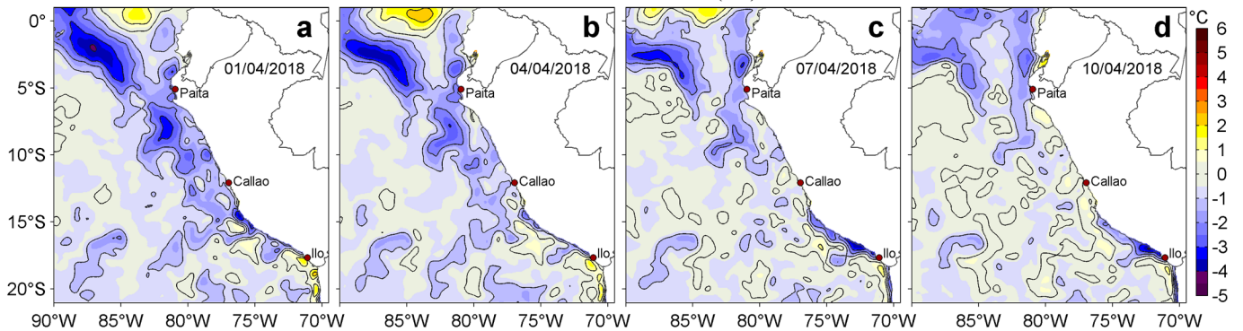
Figura 3. Anomalías de la Temperatura Superficial del Mar ( ^{\circ}\text{C} ) para los días: a) 01, b) 04, c) 07 y d) 10 de abril de 2018. Las anomalías se calcularon respecto de la climatología para el periodo 2007-2016. Datos: OSTIA-UKMO-L4-GLOB-v2.0 (UK Met Office, 2012; Donlon et al, 2012). Procesamiento: LHF/AFIOF/DGIOCC/IMARPE.
