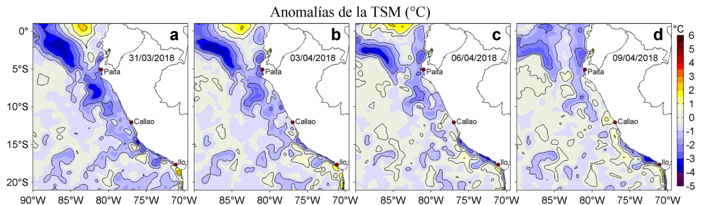
Figura 3. Anomalías de la Temperatura Superficial del Mar (°C) para los días: a) 31 de marzo, b) 03, c) 06 y d) 09 de abril de 2018. Las anomalías se calcularon respecto de la climatología para el periodo 2007-2016. Datos: OSTIA-UKMO-L4-GLOB-v2.0 (UK Met Office, 2012; Donlon et al, 2012). Procesamiento: LHF/AFIOF/DGIOCC/IMARPE.
