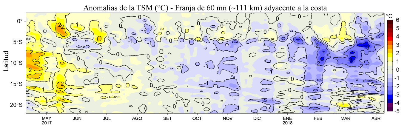
Figura 4. Variación promedio de las anomalías de la Temperatura Superficial del Mar (°C) para una franja de 60 mn (~111 km) adyacente al litoral peruano para los últimos doce meses al 09 de abril de 2018. Datos: OSTIA-UKMO-L4-GLOB-v2.0 (UK Met. Office, 2012; Donlon et al, 2012) disponible en https://podaac.jpl.nasa.gov/dataset/OSTIA-UKMO-L4-GLOB-v2.0 . Las anomalías se calcularon con respecto al periodo 2007-2016. Procesamiento: LHF/AFIOF/DGIOCC/IMARPE.
