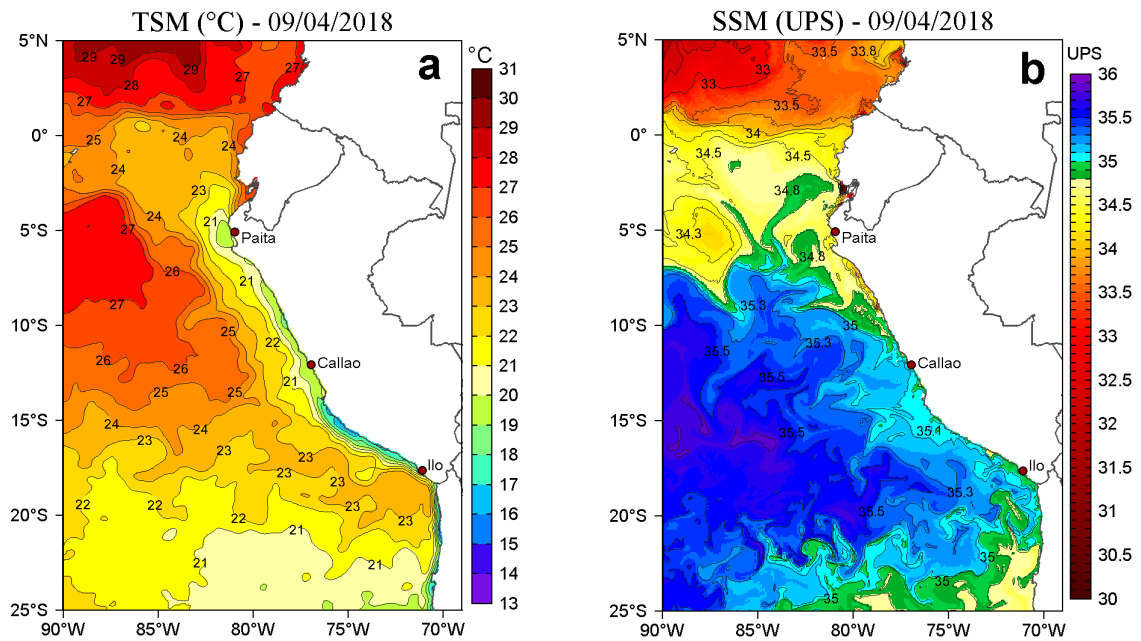
Figura 2. a) Temperatura Superficial del Mar (°C) y b) Salinidad Superficial del Mar (UPS) para el 09 de abril de 2018. Datos: OSTIA-UKMO-L4-GLOB-v2.0 (UK Met Office, 2012; Donlon et al, 2012) disponible en https://podaac.jpl.nasa.gov/dataset/OSTIA-UKMO-L4-GLOB-v2.0 para (a) y Hybrid Coordinate Ocean Model (HYCOM; Halliwell et al., 1998; 2000; Bleck, 2001) para (b). Procesamiento: LHF/AFIOF/DGIOCC/IMARPE.
