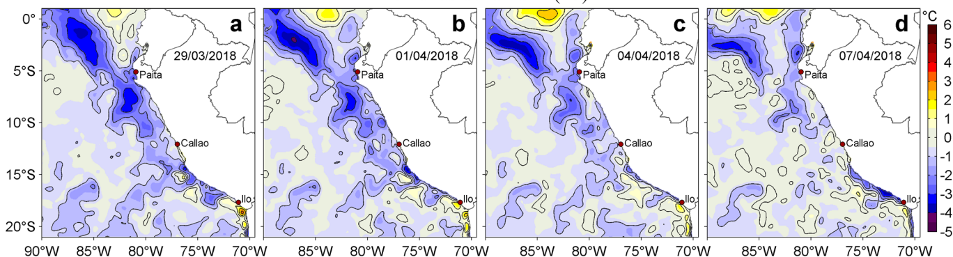
Figura 3. Anomalías de la Temperatura Superficial del Mar (°C) para los días: a) 29 de marzo, b) 01, c) 04 y d) 07 de abril de 2018. Las anomalías se calcularon respecto de la climatología para el periodo 2007-2016. Datos: OSTIA-UKMO-L4-GLOB-v2.0 (UK Met Office, 2012; Donlon et al, 2012). Procesamiento: LHF/AFIOF/DGIOCC/IMARPE.
