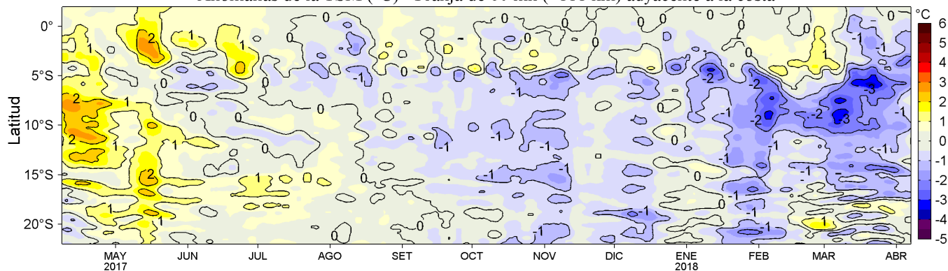
Figura 4. Variación promedio de las anomalías de la Temperatura Superficial del Mar (°C) para una franja de 60 mn (~111 km) adyacente al litoral peruano para los últimos doce meses al 07 de abril de 2018. Datos: OSTIA-UKMO-L4-GLOB-v2.0 (UK Met. Office, 2012; Donlon et al, 2012) disponible en https://podaac.jpl.nasa.gov/dataset/OSTIA-UKMO-L4-GLOB-v2.0 . Las anomalías se calcularon con respecto al periodo 2007-2016. Procesamiento: LHF/AFIOF/DGIOCC/IMARPE.
