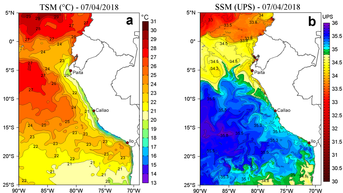
Figura 2. a) Temperatura Superficial del Mar (°C) y b) Salinidad Superficial del Mar (UPS) para el 07 de abril de 2018. Datos: OSTIA-UKMO-L4-GLOB-v2.0 (UK Met Office, 2012; Donlon et al, 2012) disponible en https://podaac.jpl.nasa.gov/dataset/OSTIA-UKMO-L4-GLOB-v2.0 para (a) y Hybrid Coordinate Ocean Model (HYCOM; Halliwell et al., 1998; 2000; Bleck, 2001) para (b). Procesamiento: LHF/AFIOF/DGIOCC/IMARPE.
