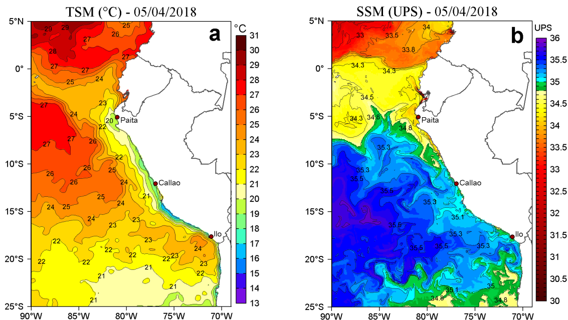
Figura 2. a) Temperatura Superficial del Mar ( ^{\circ}\text{C} ) y b) Salinidad Superficial del Mar (UPS) para el 05 de abril de 2018. Datos: OSTIA-UKMO-L4-GLOB-v2.0 (UK Met Office, 2012; Donlon et al, 2012) disponible en https://podaac.jpl.nasa.gov/dataset/OSTIA-UKMO-L4-GLOB-v2.0 para (a) y Hybrid Coordinate Ocean Model (HYCOM; Halliwell et al., 1998; 2000; Bleck, 2001) para (b). Procesamiento: LHF/AFIOF/DGIOCC/IMARPE.
