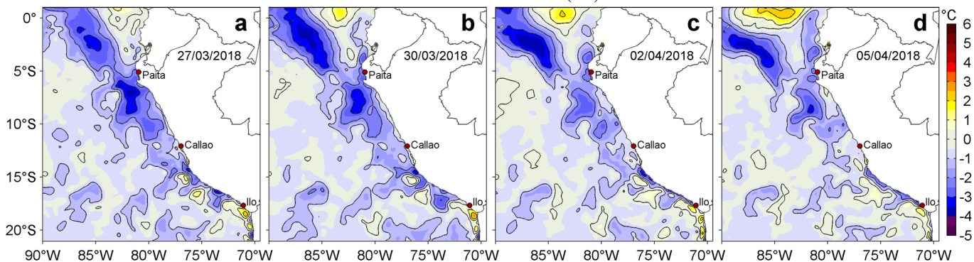
Figura 3. Anomalías de la Temperatura Superficial del Mar ( ^{\circ}\text{C} ) para los días: a) 27, b) 30 de marzo, c) 02 y d) 05 de abril de 2018. Las anomalías se calcularon respecto de la climatología para el periodo 2007-2016. Datos: OSTIA-UKMO-L4-GLOB-v2.0 (UK Met Office, 2012; Donlon et al, 2012). Procesamiento: LHF/AFIOF/DGIOCC/IMARPE.
