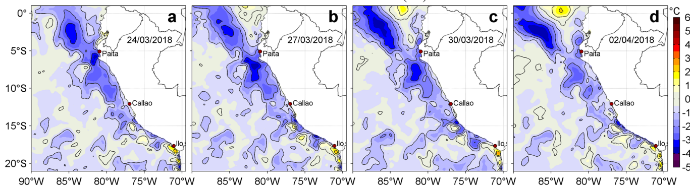
Figura 3. Anomalías de la Temperatura Superficial del Mar ( ^{\circ}\text{C} ) para los días: a) 24, b) 27, c) 30 de marzo y d) 02 de abril de 2018. Las anomalías se calcularon respecto de la climatología para el periodo 2007-2016. Datos: OSTIA-UKMO-L4-GLOB-v2.0 (UK Met Office, 2012; Donlon et al, 2012). Procesamiento: LHF/AFIOF/DGIOCC/IMARPE.
