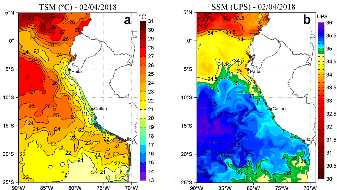
Figura 2. a) Temperatura Superficial del Mar ( ^{\circ}\text{C} ) y b) Salinidad Superficial del Mar (UPS) para el 02 de abril de 2018. Datos: OSTIA-UKMO-L4-GLOB-v2.0 (UK Met Office, 2012; Donlon et al, 2012) disponible en https://podaac.jpl.nasa.gov/dataset/OSTIA-UKMO-L4-GLOB-v2.0 para (a) y Hybrid Coordinate Ocean Model (HYCOM; Halliwell et al., 1998; 2000; Bleck, 2001) para (b). Procesamiento: LHF/AFIOF/DGIOCC/IMARPE.
