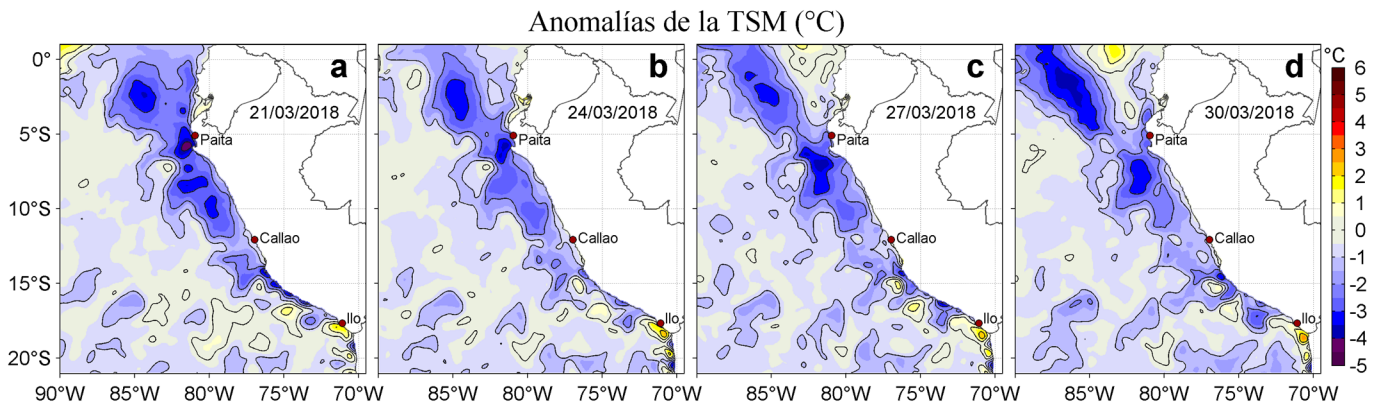
Figura 3. Anomalías de la Temperatura Superficial del Mar ( ^{\circ}\text{C} ) para los días: a) 21, b) 24, c) 27 y d) 30 de marzo de 2018. Las anomalías se calcularon respecto de la climatología para el periodo 2007-2016. Datos: OSTIA-UKMO-L4-GLOB-v2.0 (UK Met Office, 2012; Donlon et al, 2012). Procesamiento: LHF/AFIOF/DGIOCC/IMARPE.
