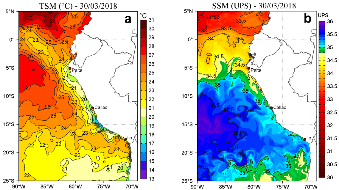
Figura 2. a) Temperatura Superficial del Mar ( ^{\circ}\text{C} ) y b) Salinidad Superficial del Mar (UPS) para el 30 de marzo de 2018. Datos: OSTIA-UKMO-L4-GLOB-v2.0 (UK Met Office, 2012; Donlon et al, 2012) disponible en https://podaac.jpl.nasa.gov/dataset/OSTIA-UKMO-L4-GLOB-v2.0 para (a) y Hybrid Coordinate Ocean Model (HYCOM; Halliwell et al., 1998; 2000; Bleck, 2001) para (b). Procesamiento: LHF/AFIOF/DGIOCC/IMARPE.
