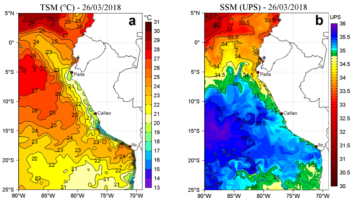
Figura 2. a) Temperatura Superficial del Mar ( ^{\circ}\text{C} ) y b) Salinidad Superficial del Mar (UPS) para el 26 de marzo de 2018. Datos: OSTIA-UKMO-L4-GLOB-v2.0 (UK Met Office, 2012; Donlon et al, 2012) disponible en https://podaac.jpl.nasa.gov/dataset/OSTIA-UKMO-L4-GLOB-v2.0 para (a) y Hybrid Coordinate Ocean Model (HYCOM; Halliwell et al., 1998; 2000; Bleck, 2001) para (b). Procesamiento: LHF/AFIOF/DGIOCC/IMARPE.
