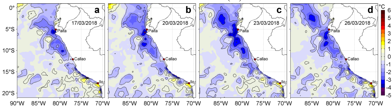
Figura 3. Anomalías de la Temperatura Superficial del Mar ( ^{\circ}\text{C} ) para los días: a) 17, b) 20, c) 23 y d) 26 de marzo de 2018. Las anomalías se calcularon respecto de la climatología para el periodo 2007-2016. Datos: OSTIA-UKMO-L4-GLOB-v2.0 (UK Met Office, 2012; Donlon et al, 2012). Procesamiento: LHF/AFIOF/DGIOCC/IMARPE.
