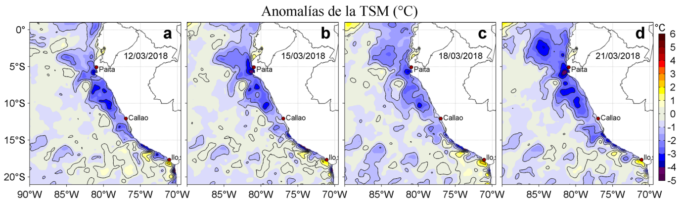
Figura 3. Anomalías de la Temperatura Superficial del Mar ( ^{\circ}\text{C} ) para los días: a) 12, b) 15, c) 18 y d) 21 de marzo de 2018. Las anomalías se calcularon respecto de la climatología para el periodo 2007-2016. Datos: OSTIA-UKMO-L4-GLOB-v2.0 (UK Met Office, 2012; Donlon et al, 2012). Procesamiento: LHF/AFIOF/DGIOCC/IMARPE.
