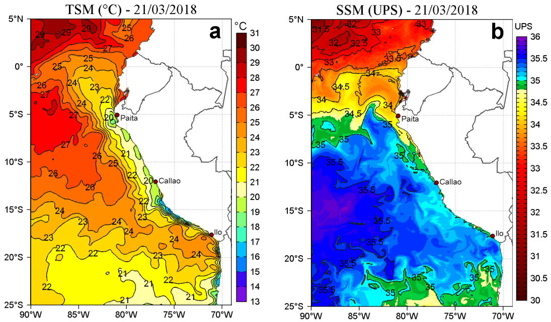
Figura 2. a) Temperatura Superficial del Mar ( ^{\circ}\text{C} ) y b) Salinidad Superficial del Mar (UPS) para el 21 de marzo de 2018. Datos: OSTIA-UKMO-L4-GLOB-v2.0 (UK Met Office, 2012; Donlon et al, 2012) disponible en https://podaac.jpl.nasa.gov/dataset/OSTIA-UKMO-L4-GLOB-v2.0 para (a) y Hybrid Coordinate Ocean Model (HYCOM; Halliwell et al., 1998; 2000; Bleck, 2001) para (b). Procesamiento: LHF/AFIOF/DGIOCC/IMARPE.
