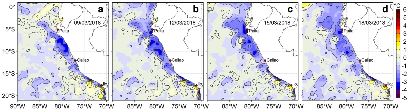
Figura 3. Anomalías de la Temperatura Superficial del Mar (°C) para los días: a) 09, b) 12, c) 15 y d) 18 de marzo de 2018. Las anomalías se calcularon respecto de la climatología para el periodo 2007-2016. Datos: OSTIA-UKMO-L4-GLOB-v2.0 (UK Met Office, 2012; Donlon et al, 2012). Procesamiento: LHFM/AFIOF/DGIOCC/IMARPE.
