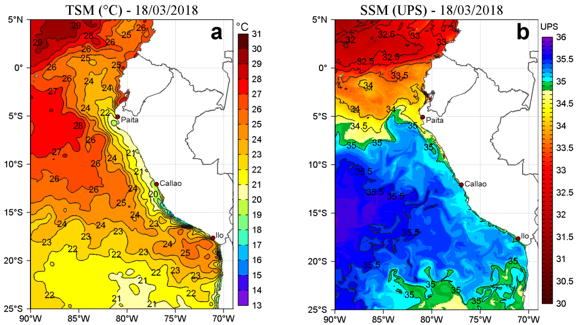
Figura 2. a) Temperatura Superficial del Mar (°C) y b) Salinidad Superficial del Mar (UPS) para el 18 de marzo de 2018. Datos: OSTIA-UKMO-L4-GLOB-v2.0 (UK Met Office, 2012; Donlon et al, 2012) disponible en https://podaac.jpl.nasa.gov/dataset/OSTIA-UKMO-L4-GLOB-v2.0 para (a) y Hybrid Coordinate Ocean Model (HYCOM; Halliwell et al., 1998; 2000; Bleck, 2001) para (b). Procesamiento: LHFM/AFIOF/DGIOCC/IMARPE.
