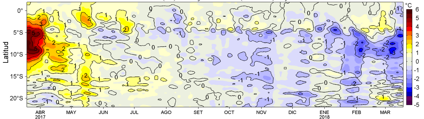
Figura 4. Variación promedio de las anomalías de la Temperatura Superficial del Mar (°C) para una franja de 60 mn (~111 km) adyacente al litoral peruano para los últimos doce meses al 18 de marzo de 2018. Datos: OSTIA-UKMO-L4-GLOB-v2.0 (UK Met. Office, 2012; Donlon et al, 2012) disponible en https://podaac.jpl.nasa.gov/dataset/OSTIA-UKMO-L4-GLOB-v2.0 ). Las anomalías se calcularon con respecto al periodo 2007-2016. Procesamiento: LHFM/AFIOF/DGIOCC/IMARPE.
