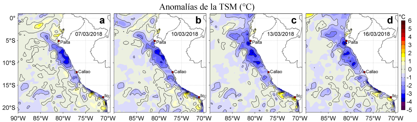
Figura 3. Anomalías de la Temperatura Superficial del Mar ( ^{\circ}\text{C} ) para los días: a) 07, b) 10, c) 13 y d) 16 de marzo de 2018. Las anomalías se calcularon respecto de la climatología para el periodo 2007-2016. Datos: OSTIA-UKMO-L4-GLOB-v2.0 (UK Met Office, 2012; Donlon et al, 2012). Procesamiento: LHF/AFIOF/DGIOCC/IMARPE.
