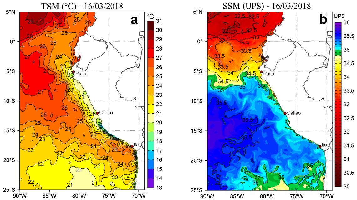
Figura 2. a) Temperatura Superficial del Mar ( ^{\circ}\text{C} ) y b) Salinidad Superficial del Mar (UPS) para el 16 de marzo de 2018. Datos: OSTIA-UKMO-L4-GLOB-v2.0 (UK Met Office, 2012; Donlon et al, 2012) disponible en https://podaac.jpl.nasa.gov/dataset/OSTIA-UKMO-L4-GLOB-v2.0 para (a) y Hybrid Coordinate Ocean Model (HYCOM; Halliwell et al., 1998; 2000; Bleck, 2001) para (b). Procesamiento: LHF/AFIOF/DGIOCC/IMARPE.
