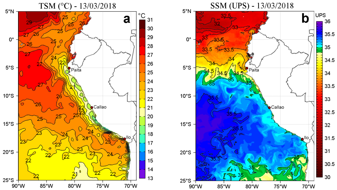
Figura 2. a) Temperatura Superficial del Mar ( ^{\circ}\text{C} ) y b) Salinidad Superficial del Mar (UPS) para el 13 de marzo de 2018. Datos: OSTIA-UKMO-L4-GLOB-v2.0 (UK Met Office, 2012; Donlon et al, 2012) disponible en https://podaac.jpl.nasa.gov/dataset/OSTIA-UKMO-L4-GLOB-v2.0 para (a) y Hybrid Coordinate Ocean Model (HYCOM; Halliwell et al., 1998; 2000; Bleck, 2001) para (b). Procesamiento: LHF/AFIOF/DGIOCC/IMARPE.
