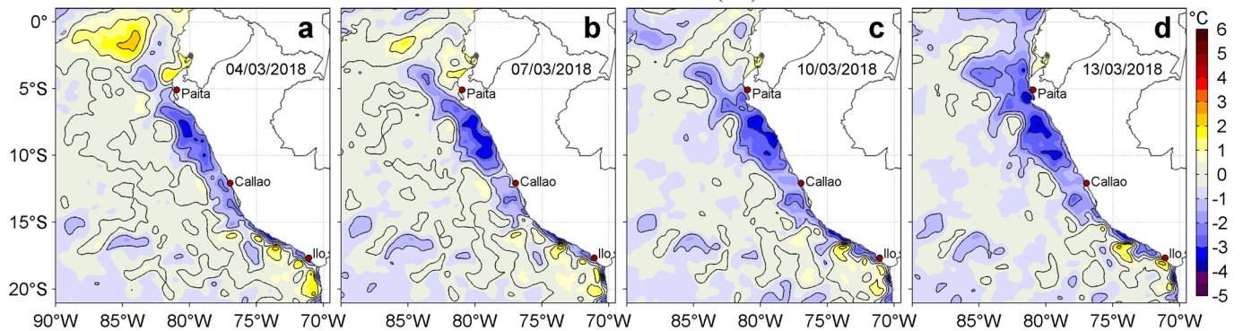
Figura 3. Anomalías de la Temperatura Superficial del Mar ( ^{\circ}\text{C} ) para los días: a) 04, b) 07, c) 10 y d) 13 de marzo de 2018. Las anomalías se calcularon respecto de la climatología para el periodo 2007-2016. Datos: OSTIA-UKMO-L4-GLOB-v2.0 (UK Met Office, 2012; Donlon et al, 2012). Procesamiento: LHF/AFIOF/DGIOCC/IMARPE.
